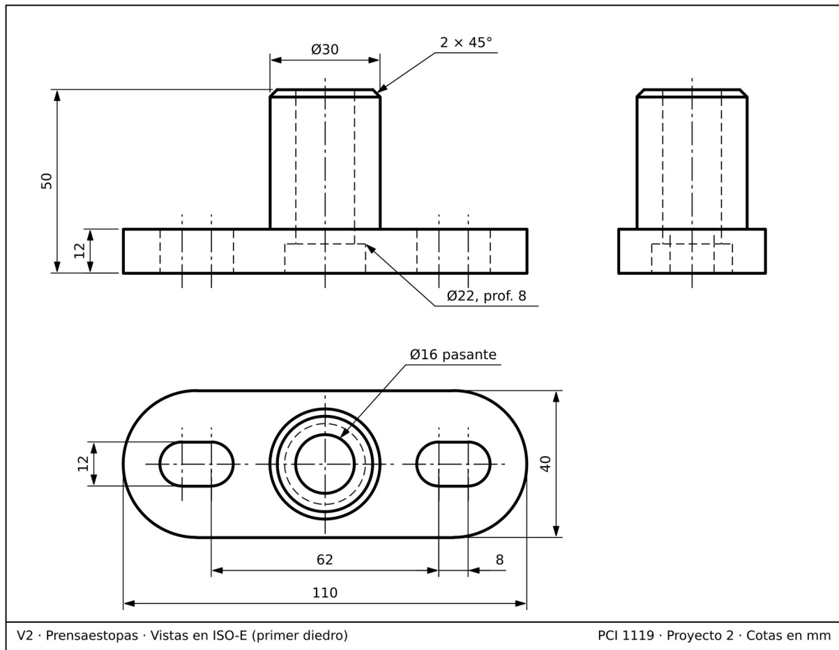
Figura 3. V2 Prensaestopas, vistas acotadas.
