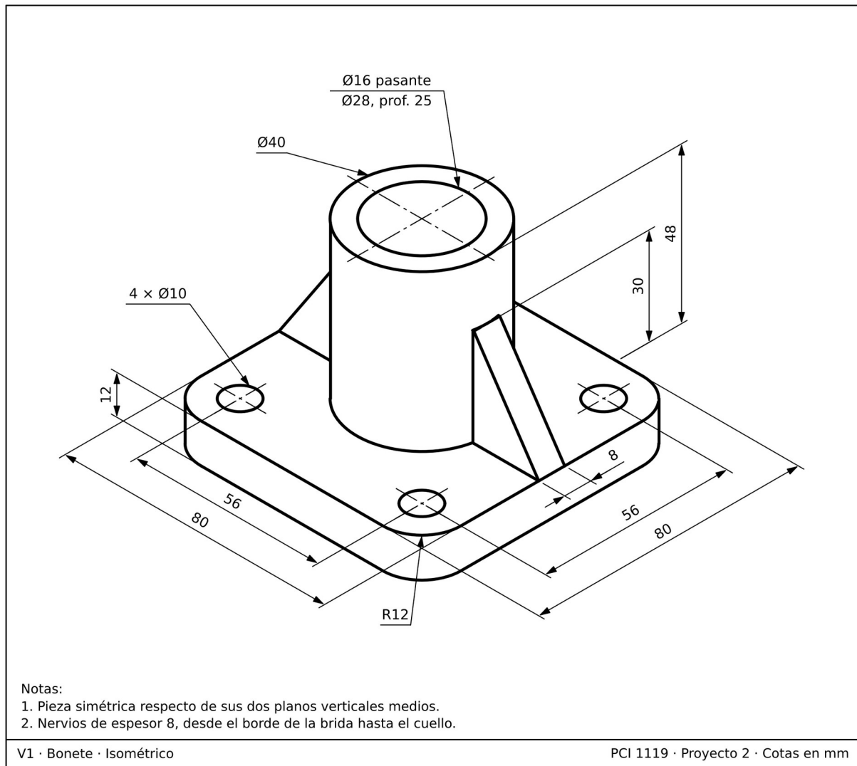
Figura 2. V1 Bonete, isométrico acotado.
