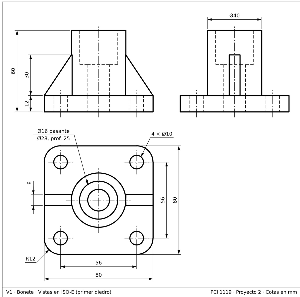
Figura 1. V1 Bonete, vistas acotadas.
