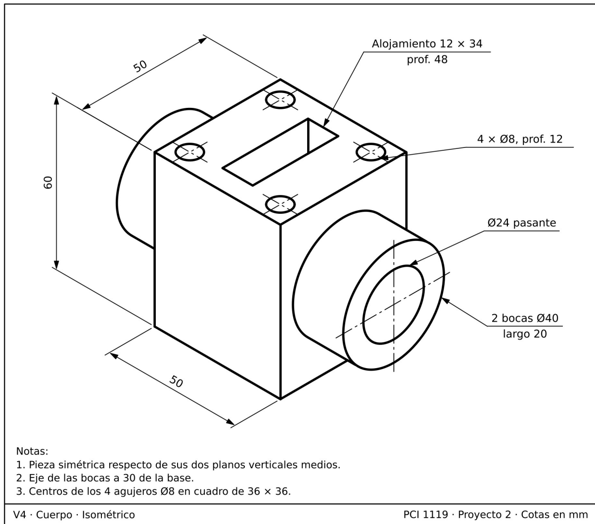
Figura 8. V4 Cuerpo, isométrico acotado.
