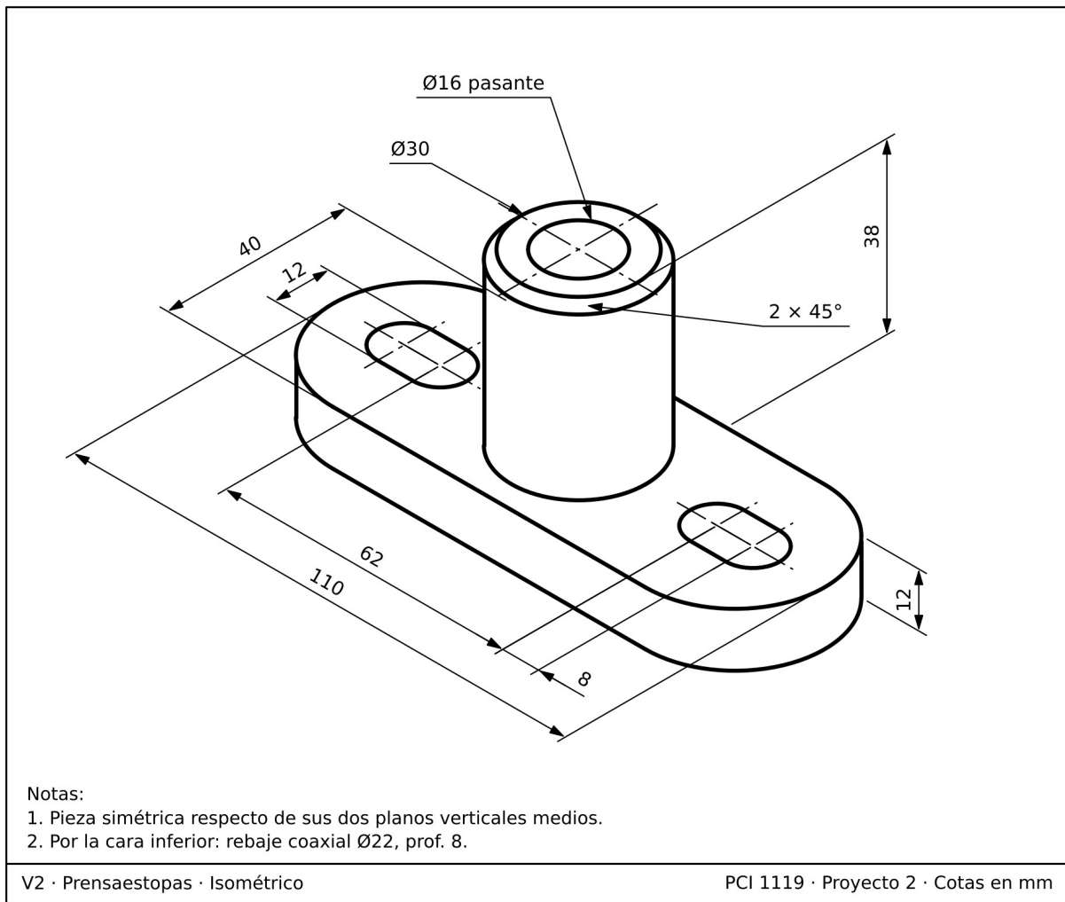
Figura 4. V2 Prensaestopas, isométrico acotado.
