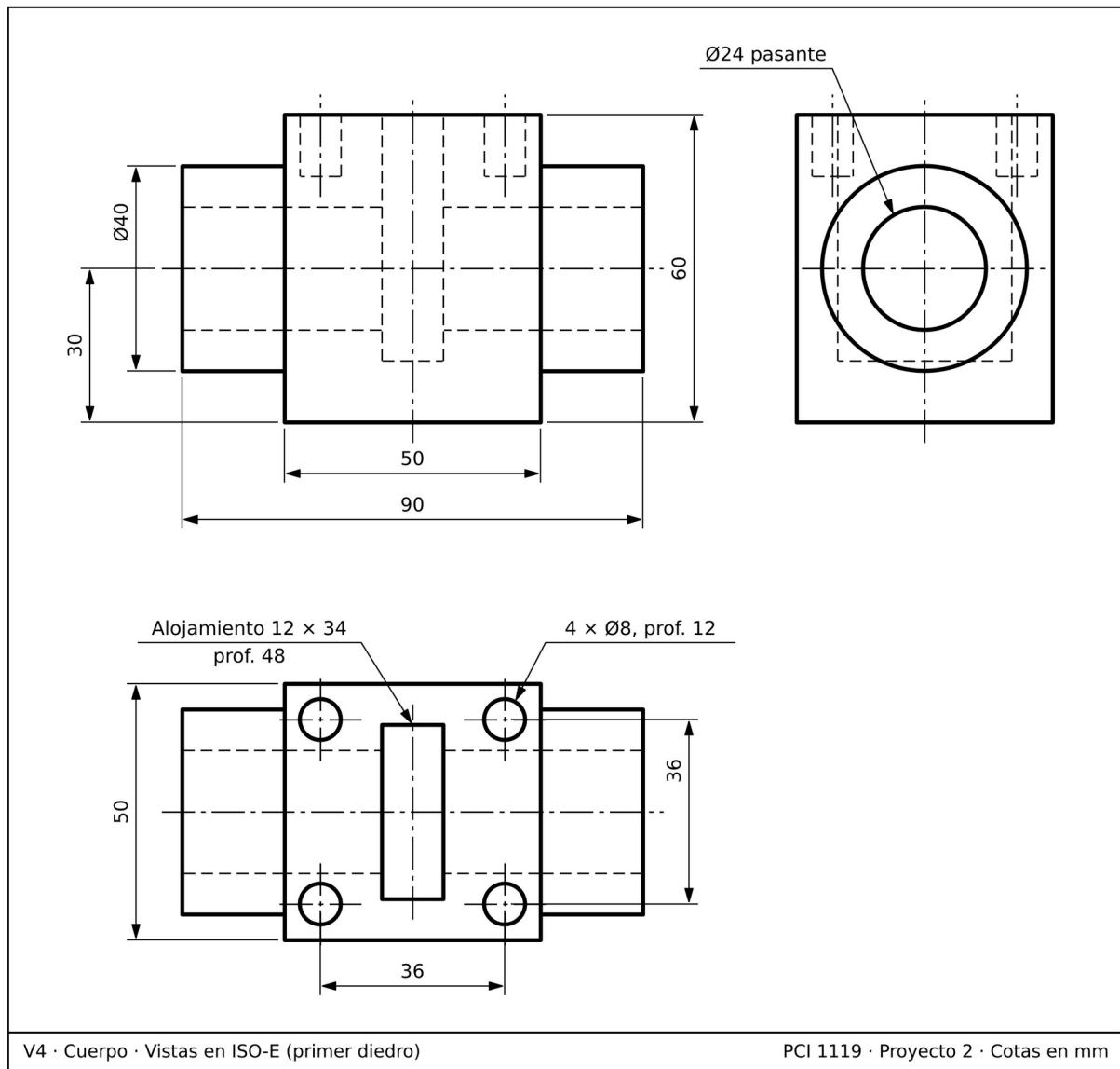
Figura 7. V4 Cuerpo, vistas acotadas.
