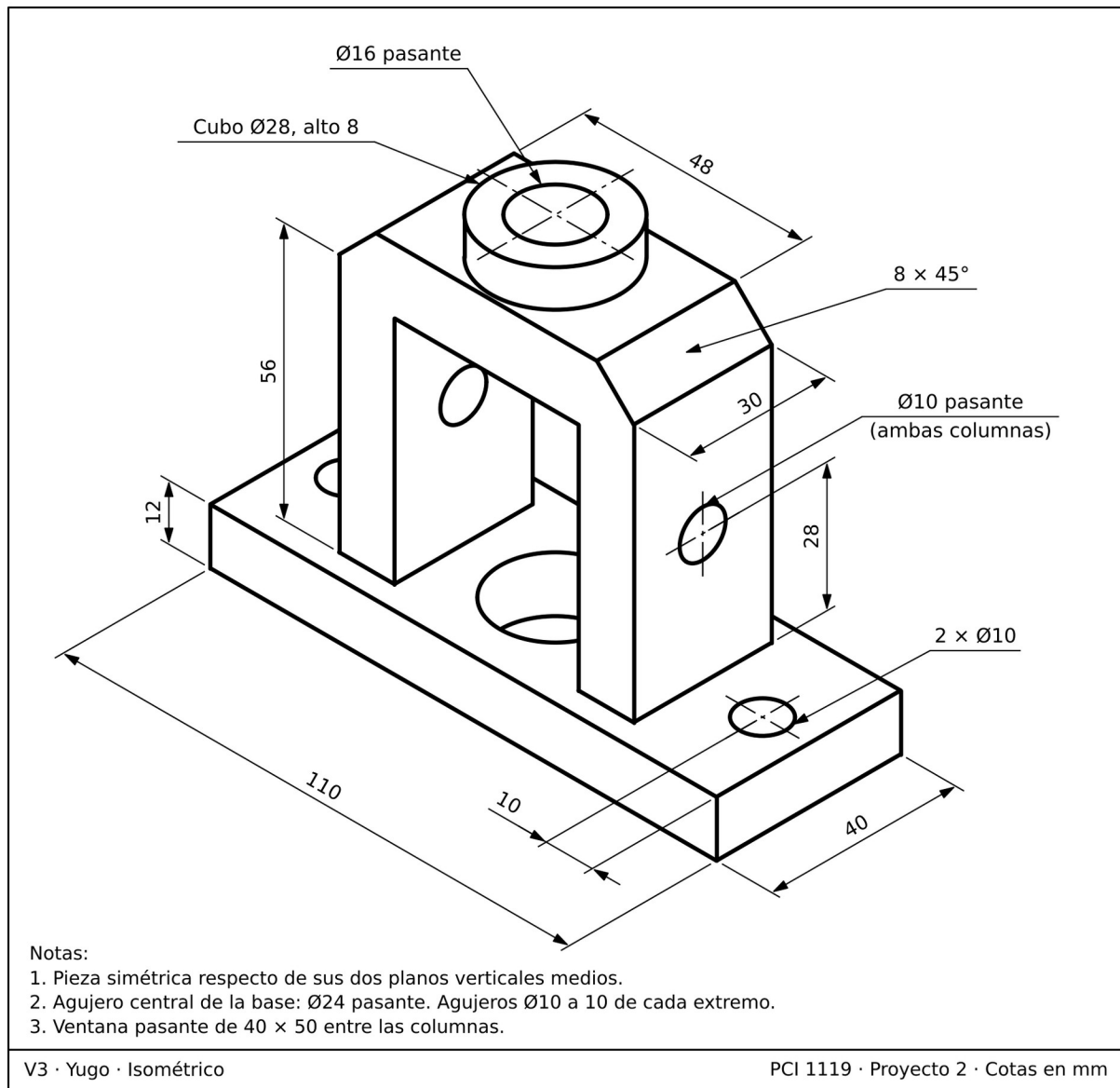
Figura 6. V3 Yugo, isométrico acotado.
