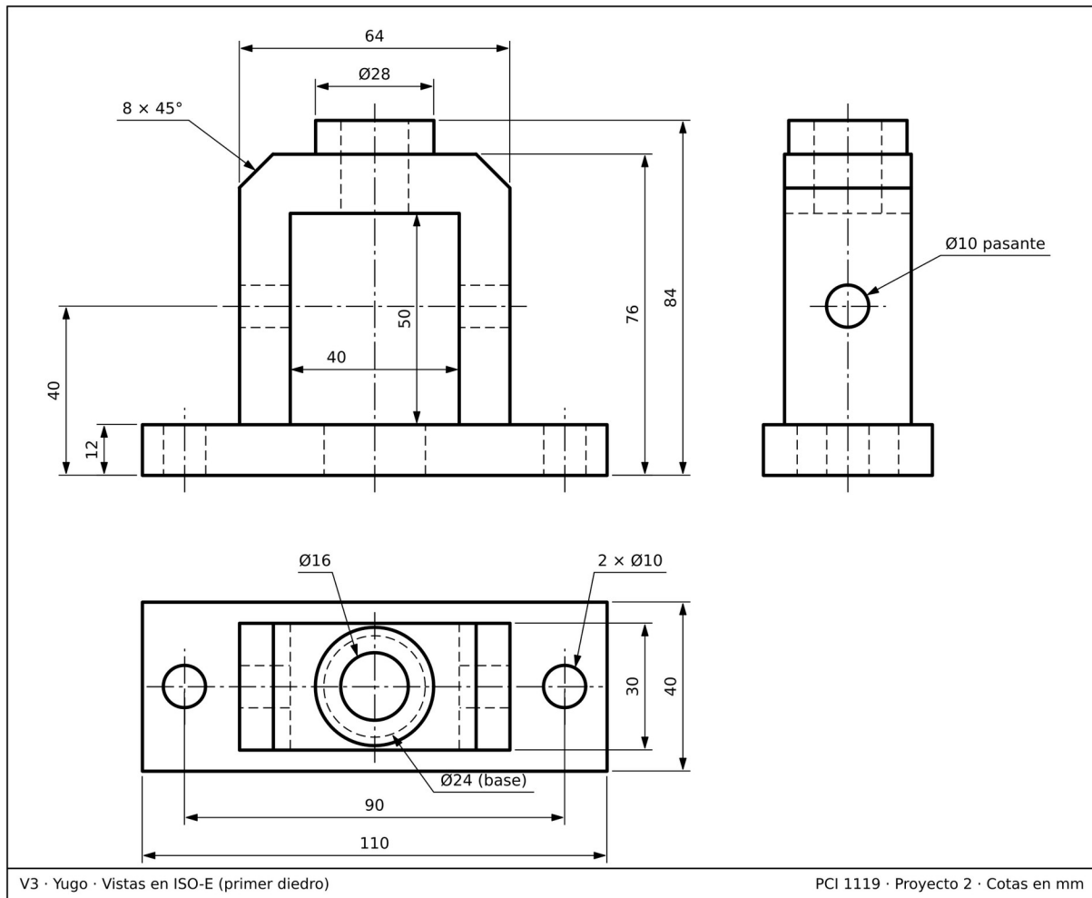
Figura 5. V3 Yugo, vistas acotadas.
