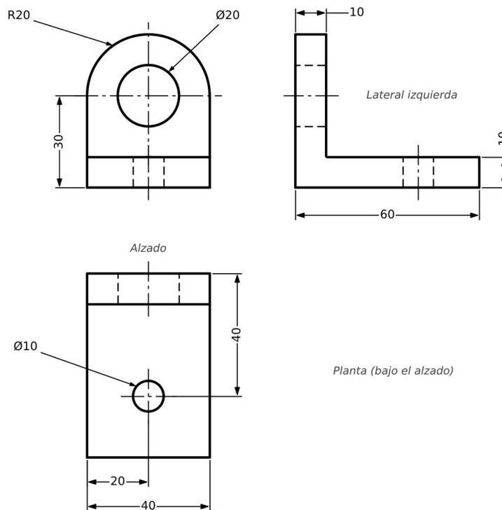
Figura 3. Soporte con respaldo redondeado.
