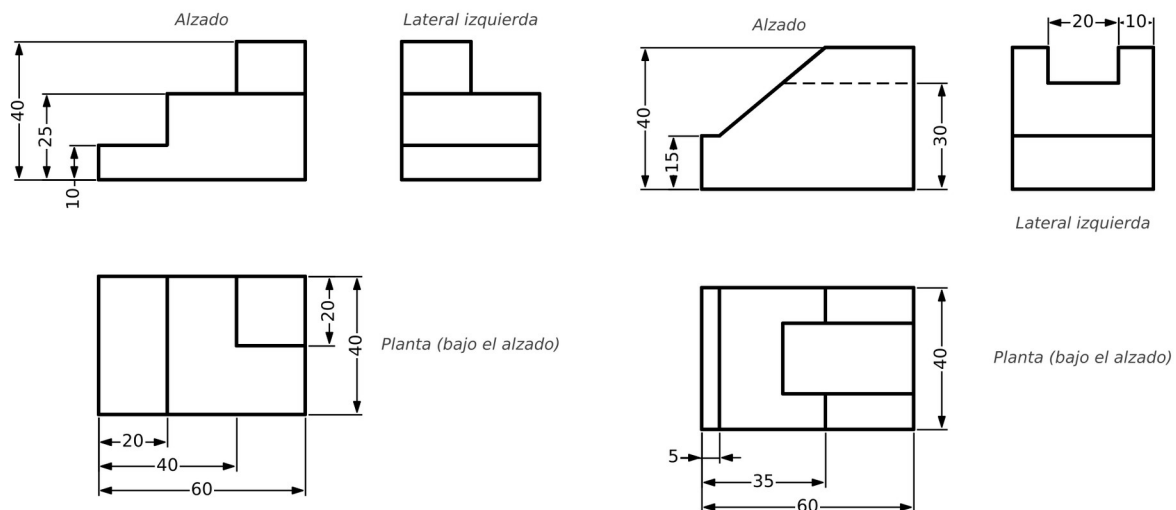
Figura 1. Pieza escalonada (izquierda). Figura 2. Pieza con plano inclinado (derecha).
