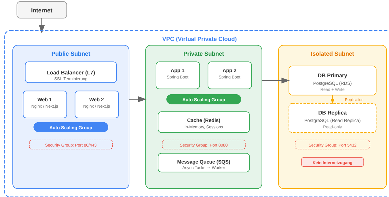
3-Tier in der Cloud
