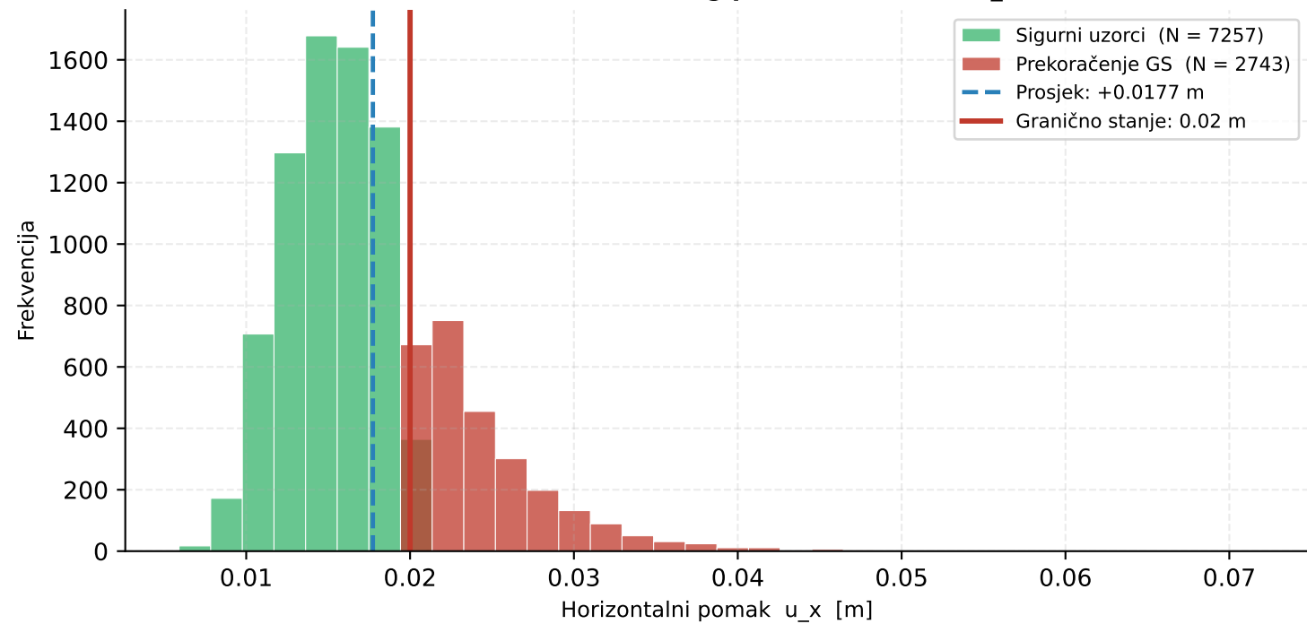
Razdioba horizontalnog pomaka čvora 2 ( u_x )
