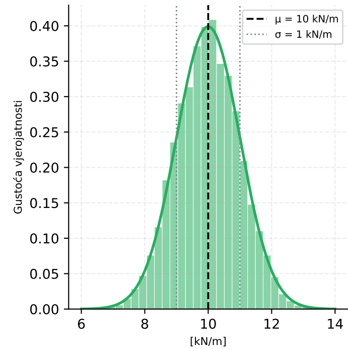
Raspodijeljeno opterećenje q
