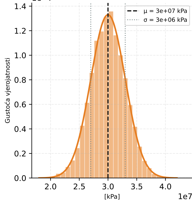
Modul elastičnosti E
