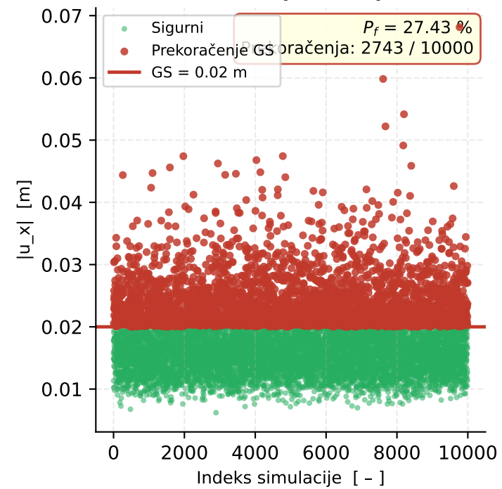
MC uzorci — apsolutni pomak
