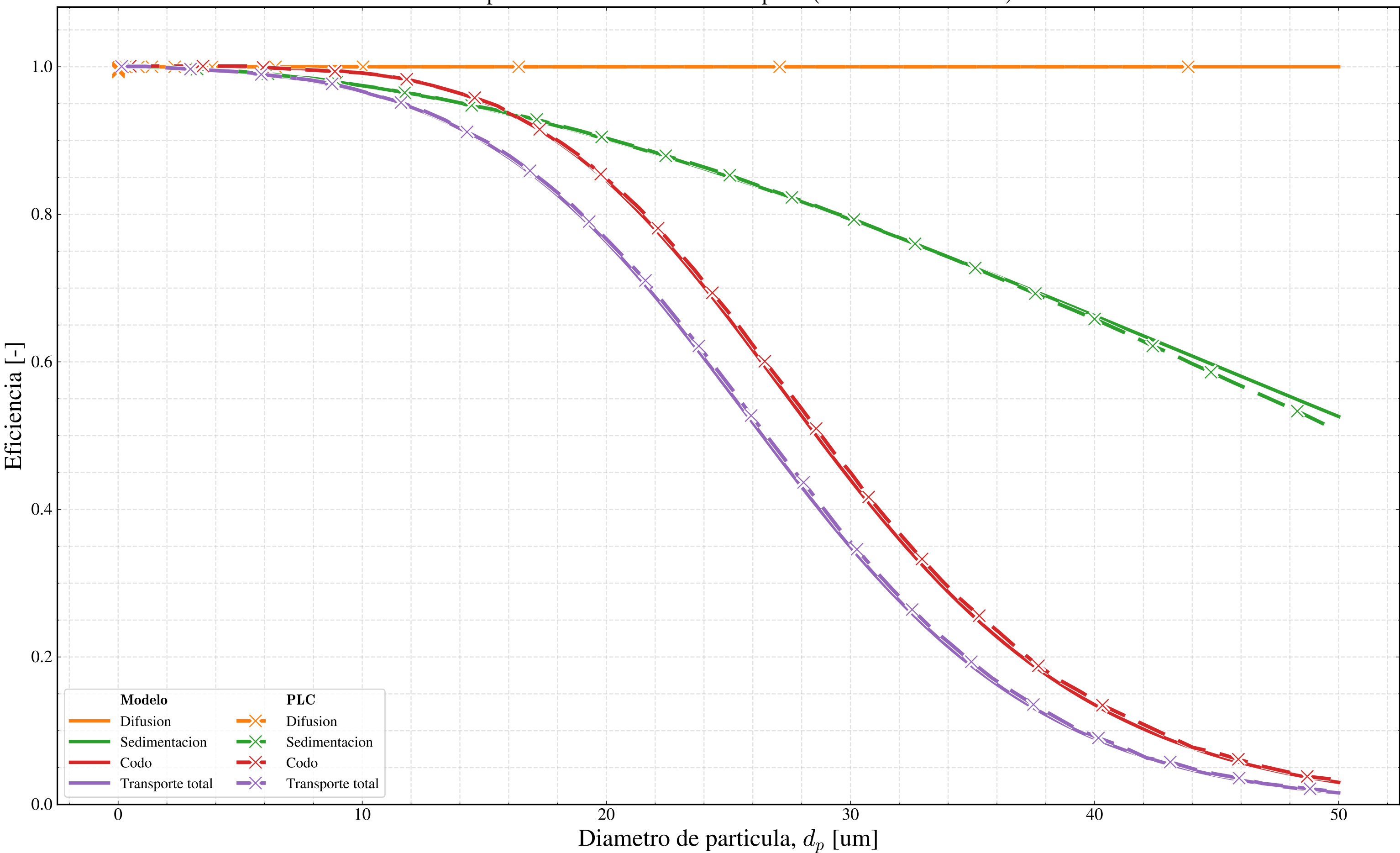
Comparacion de eficiencias de transporte (Modelo vs PLC New)
