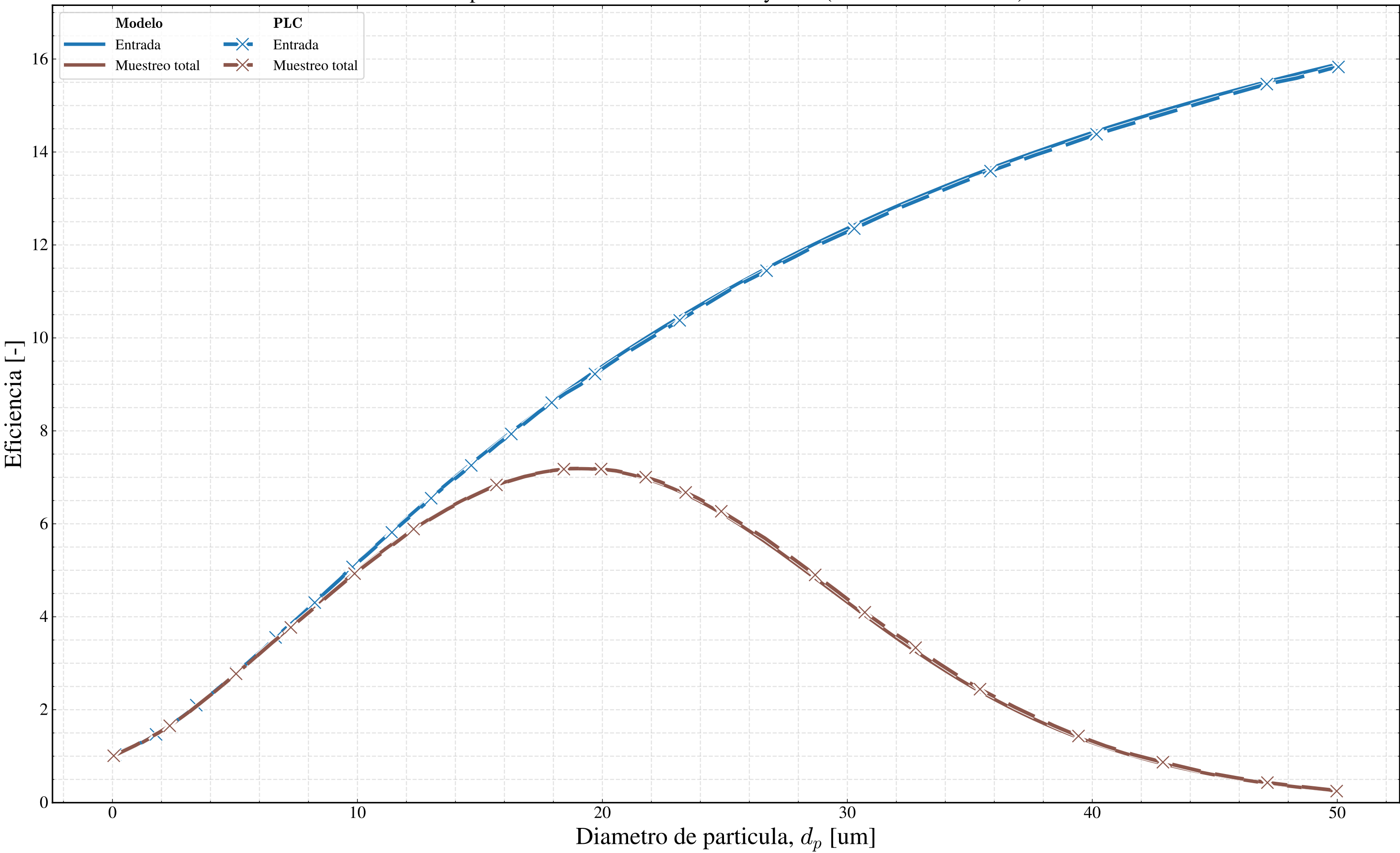
Comparacion de eficiencia de entrada y total (Modelo vs PLC New)
