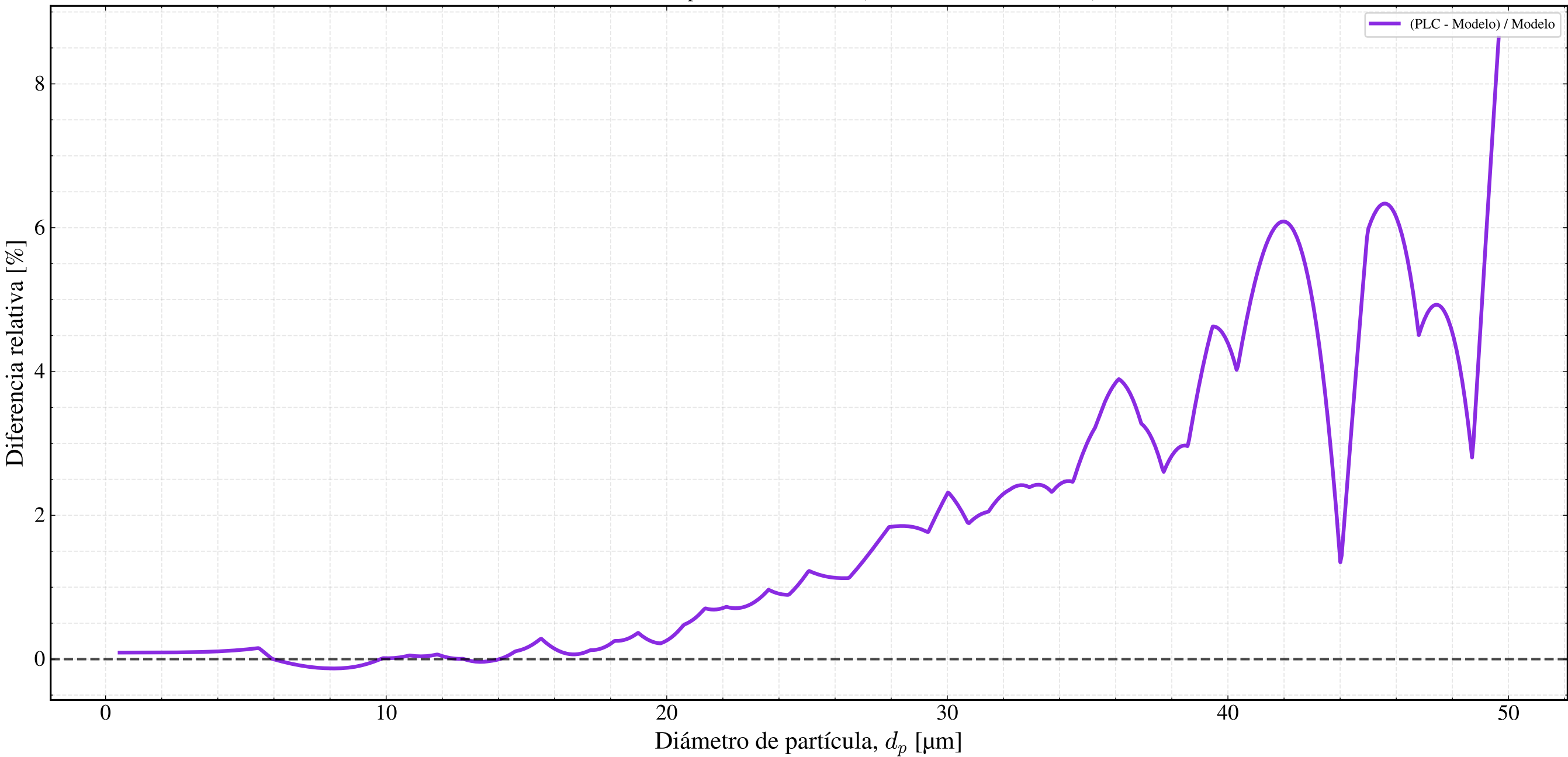
Diferencia relativa porcentual de codo ( 0^\circ + 60^\circ , PLC vs Modelo)
