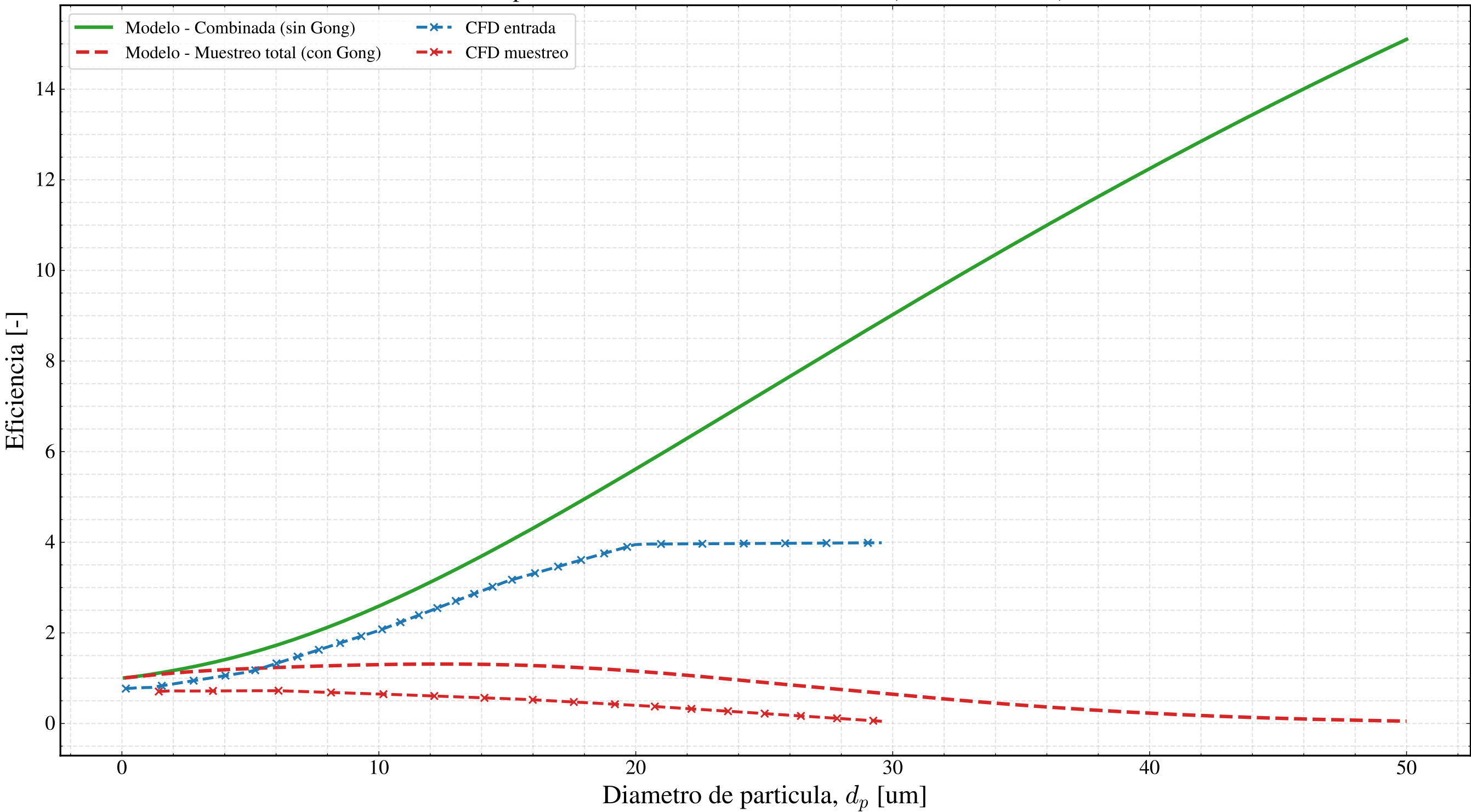
Comparacion de eficiencias seleccionadas (Modelo vs CFD)
