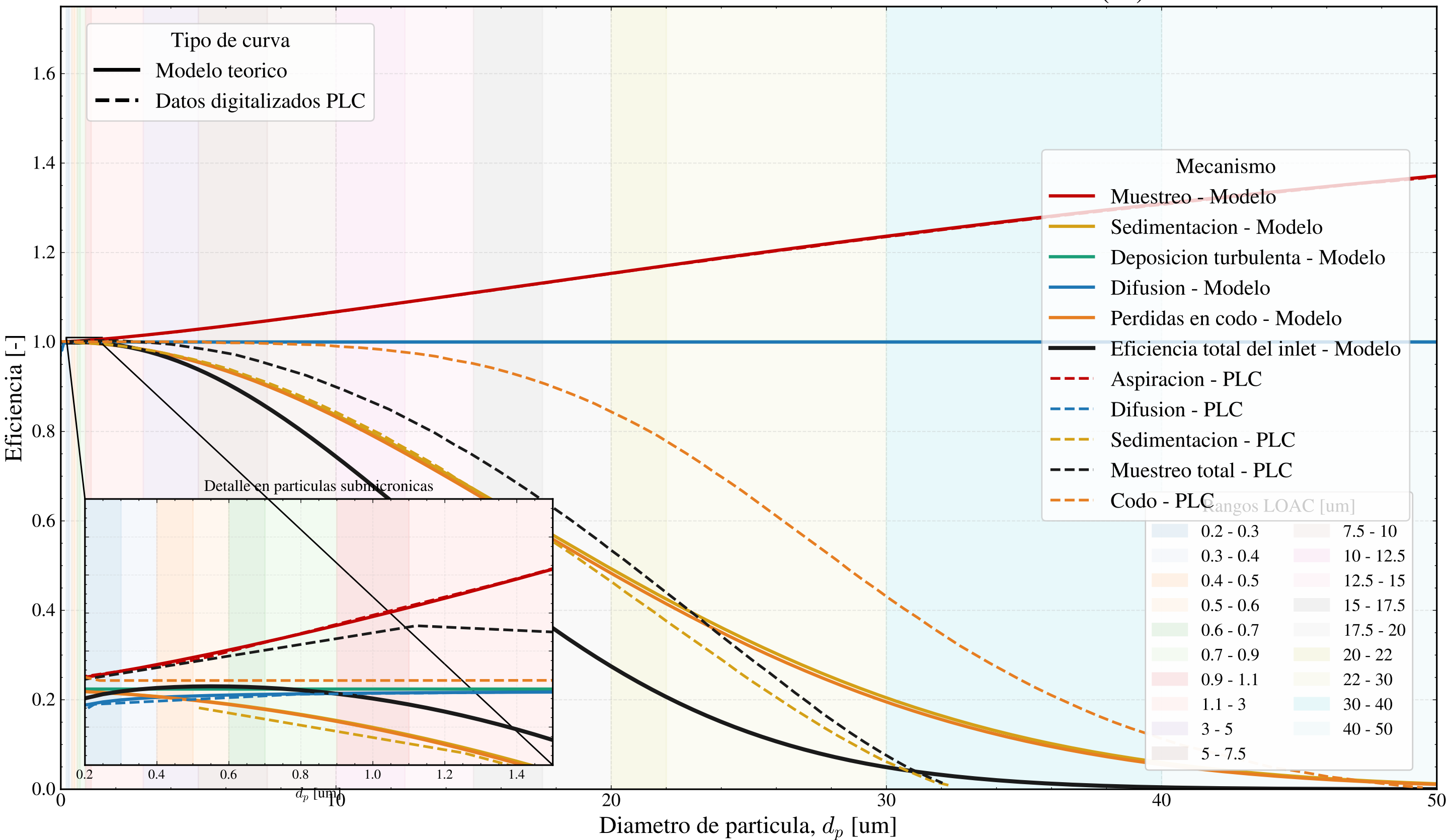
Validación del metodo de eficiencia del inlet frente a resultados PLC (v2)
