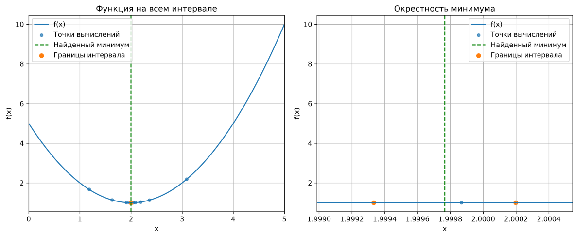
Рис. 4. Метод золотого сечения на функции f_1 .
