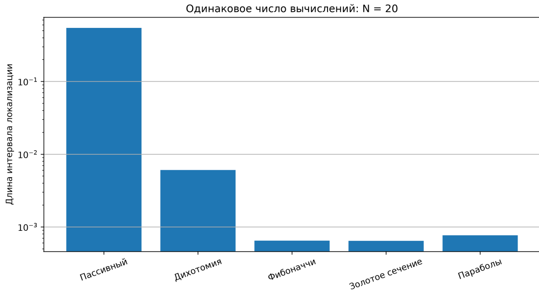
Рис. 17. Сравнение длины итогового интервала при одинаковом числе вычислений.
