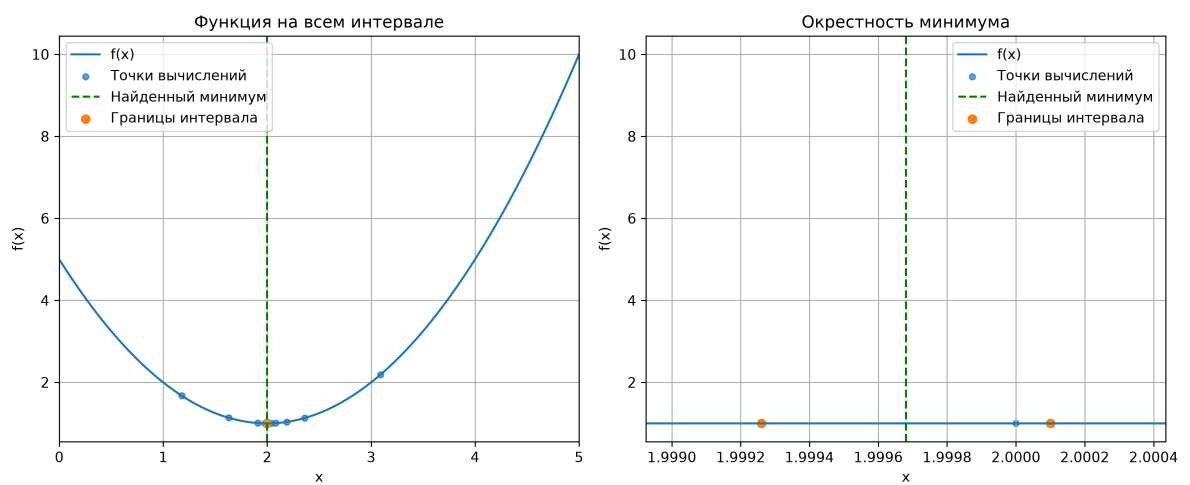
Рис. 3. Метод Фибоначчи на функции f_1 .
