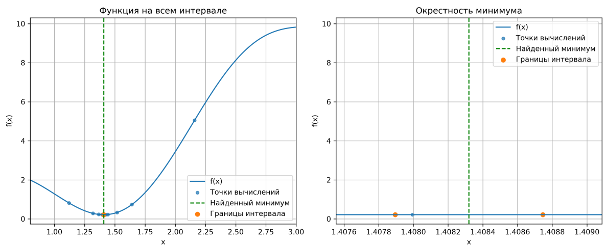
Рис. 8. Метод Фибоначчи на функции f_2 .
