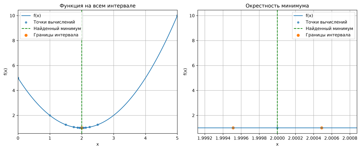
Рис. 5. Метод парабол на функции f_1 .
