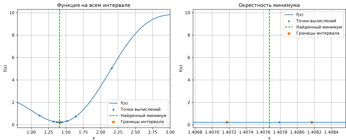
Рис. 9. Метод золотого сечения на функции f_2 .
