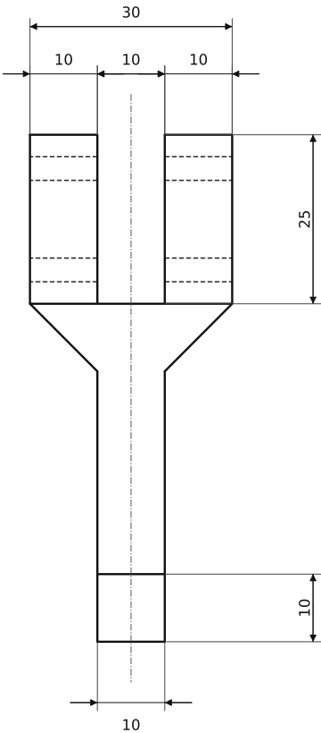
VISTA LATERAL
