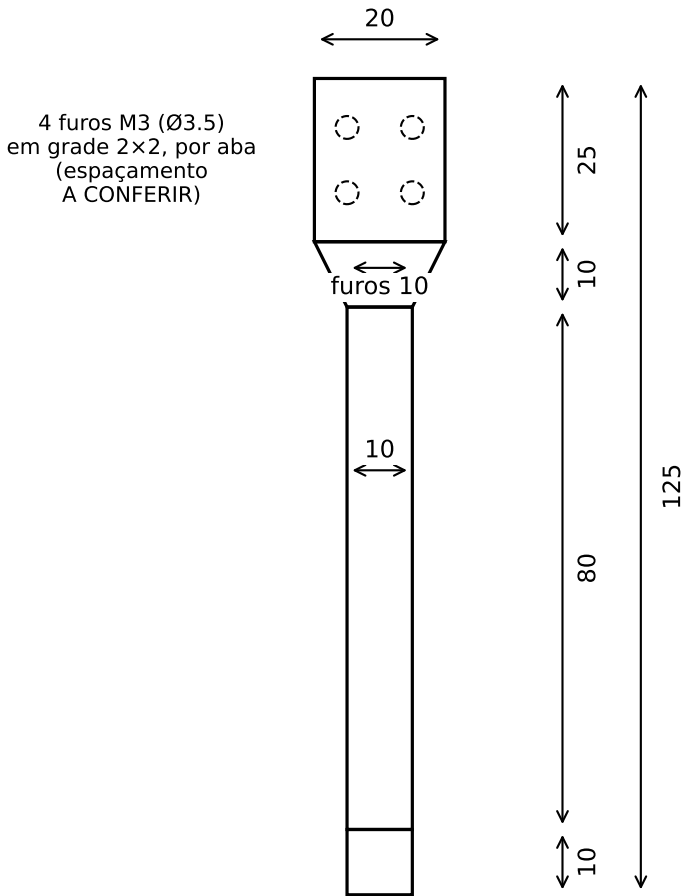
Vista de frente (X-Z) — o degrau visto de ponta
