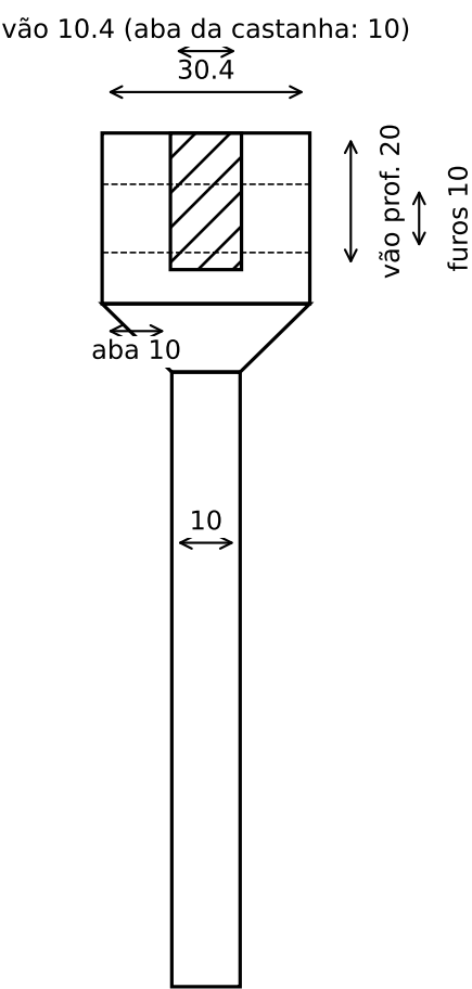
Vista lateral (Y-Z) — o U do garfo e a seção 10 × 10
