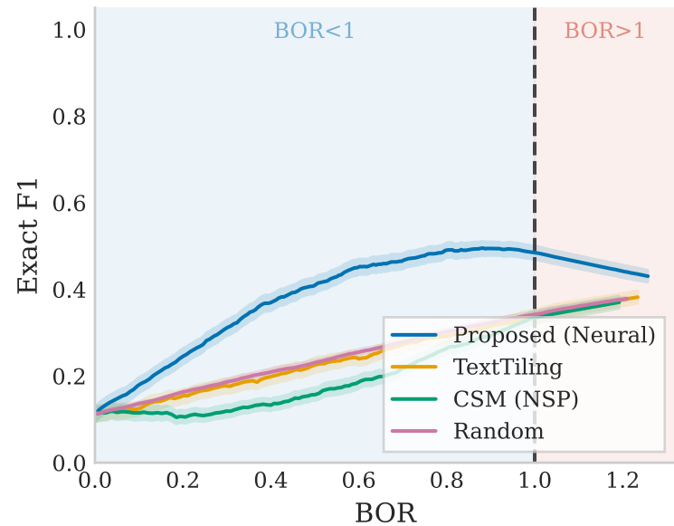
Exact F1
