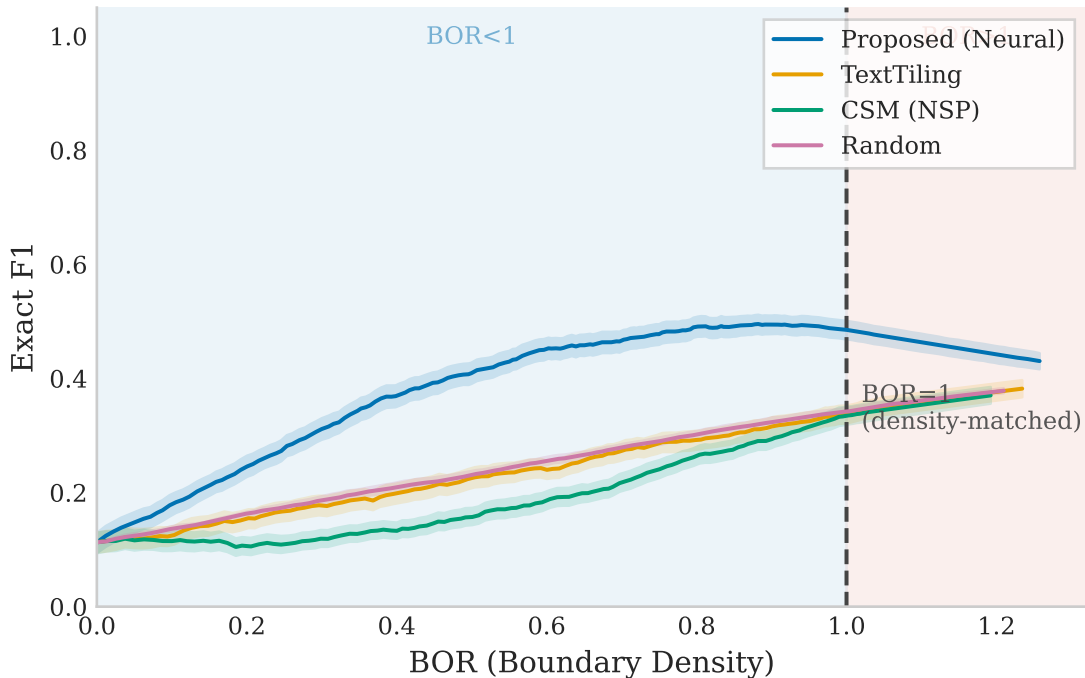
SuperSeg: Exact F1 vs Boundary Density
