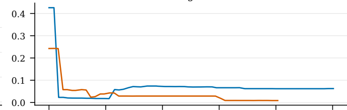
D3 alg conn
