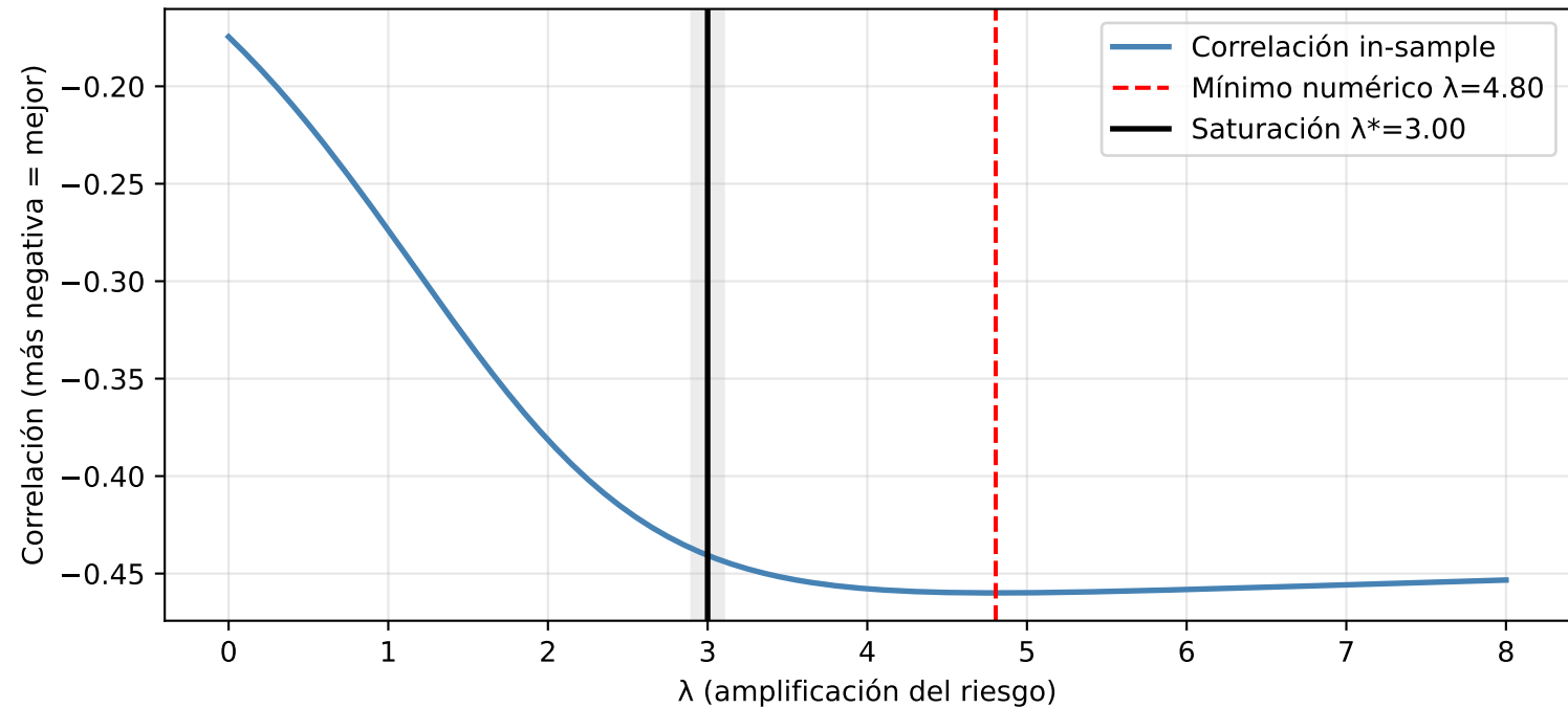
Curva de correlación con crecimiento t+1 en función de \lambda
