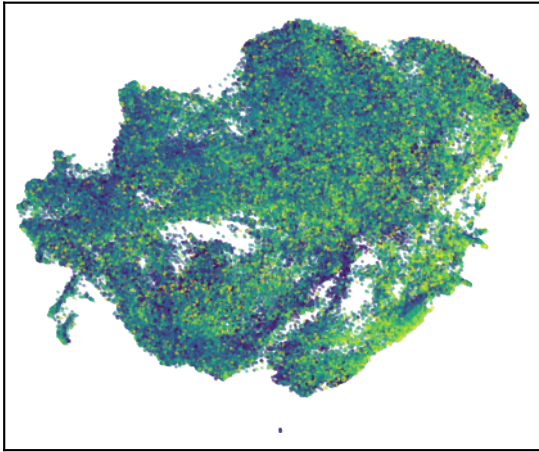
P(late disk)
