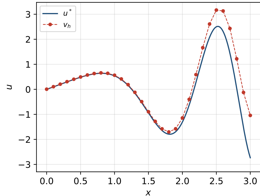
схема O(h^1) , n = 30
