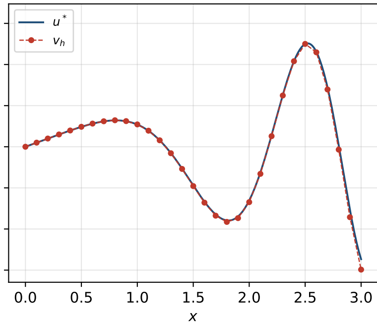
схема O(h^2) , n = 30
