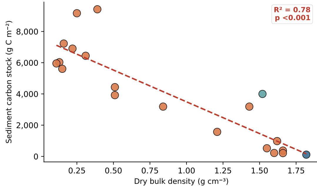
A. Dry Bulk Density
