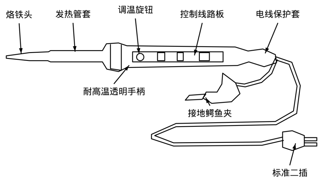
(c) 调温电烙铁结构
