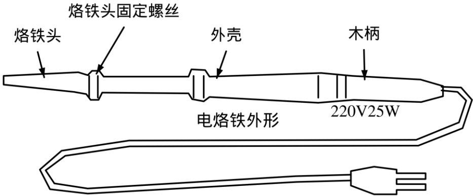
(b) 外热式电烙铁结构
