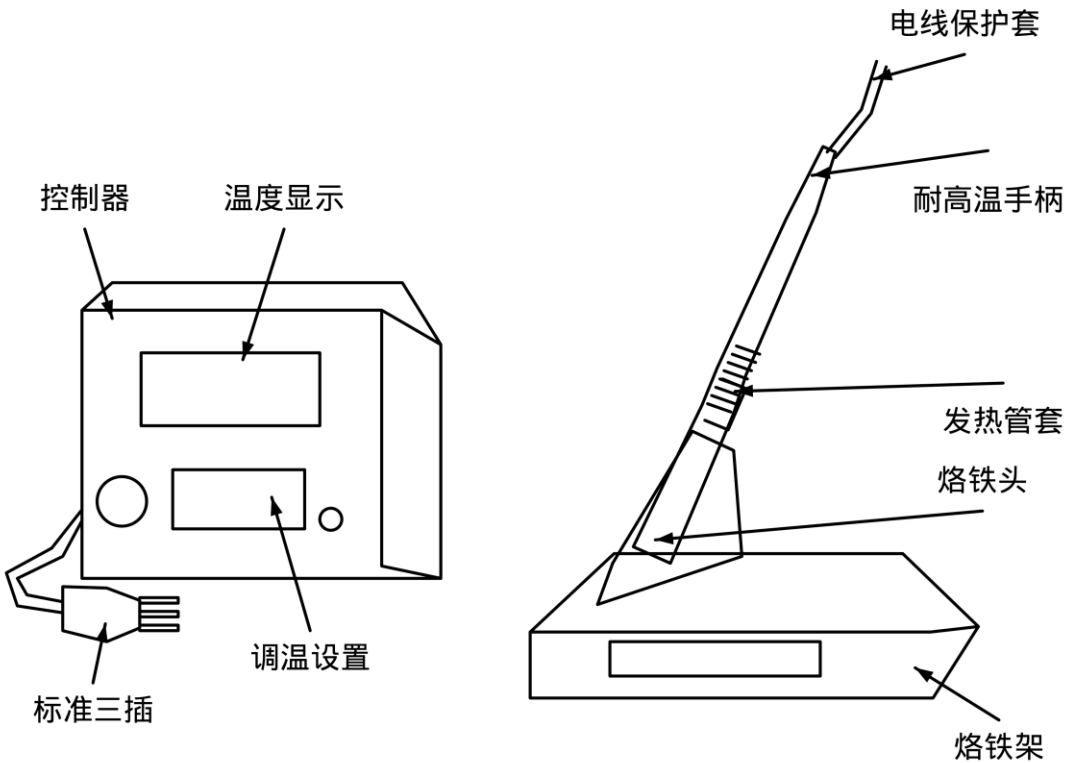
(c) 调温电烙铁结构
