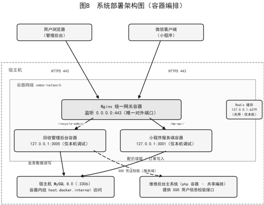
图 2-2 系统总体部署架构图
