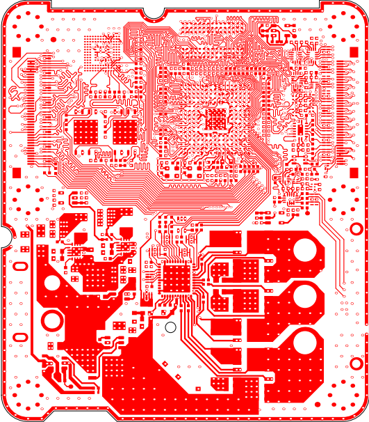
SIG1 (Scale 1:1)
