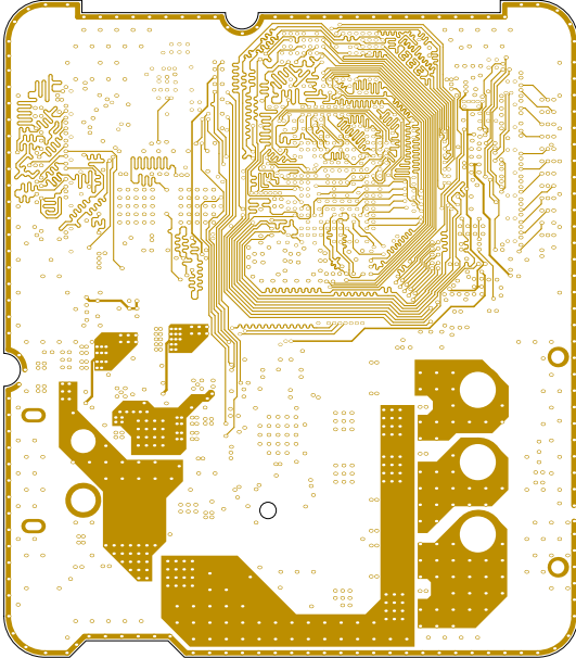
SIG3 (Scale 1:1)
