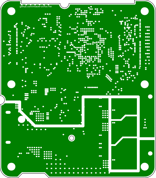
GND2 (Scale 1:1)
