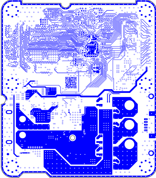
SIG6 (Scale 1:1)
