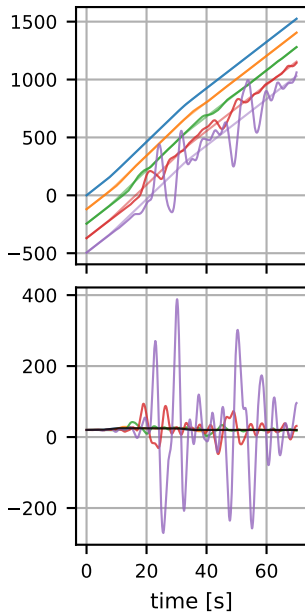
Linear feedback
