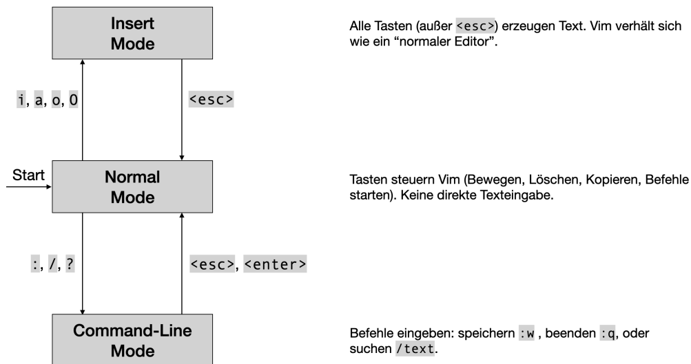
Abbildung 1: Zustandsdiagramm der drei wichtigsten Vim-Modi: Normal, Insert und Command-Line.
