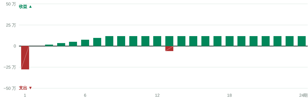
图 5-3 24 期收支分布
