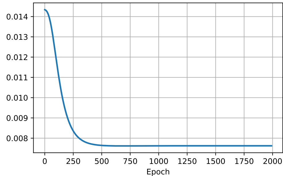
Phi Matrix Error (MSE)
