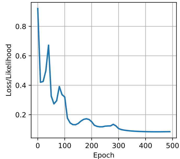
AR Error
