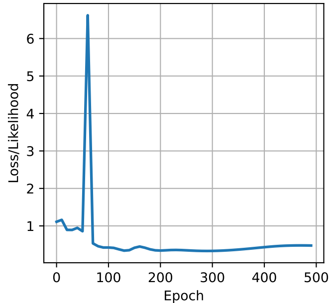
AR Error
