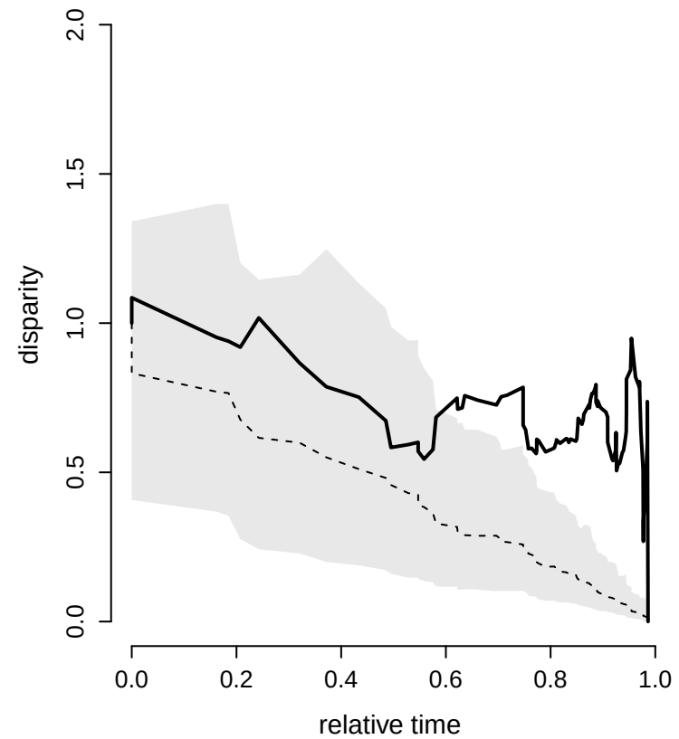
PC3 (MDI = 0.3360)
