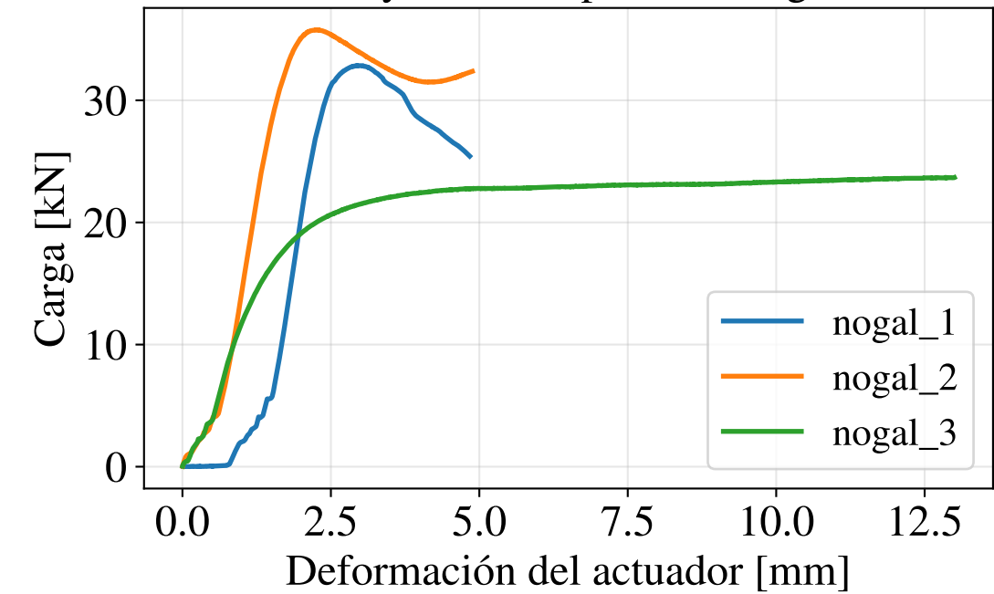
Ensayos de compresión: Nogal
