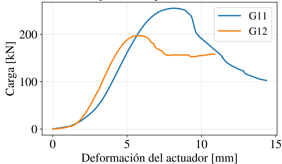
Ensayos de compresión: Guadua 1
