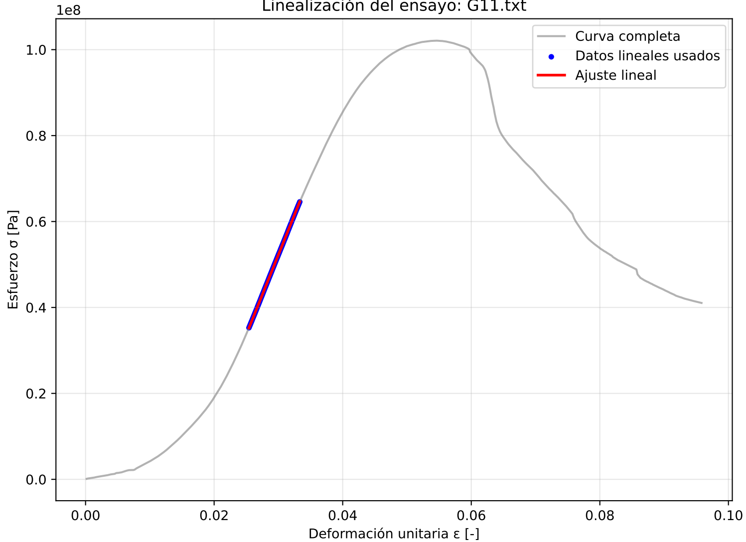
Linealización del ensayo: G11.txt
