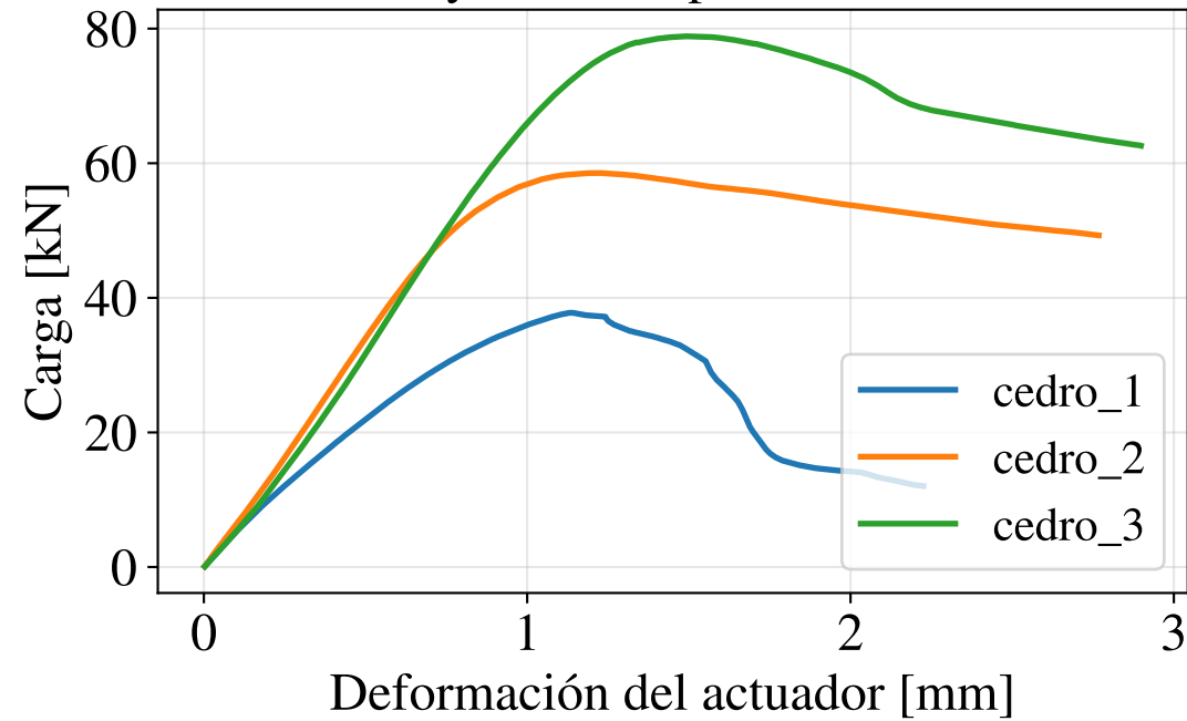
Ensayos de compresión: Cedro
