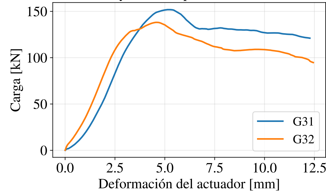
Ensayos de compresión: Guadua 3
