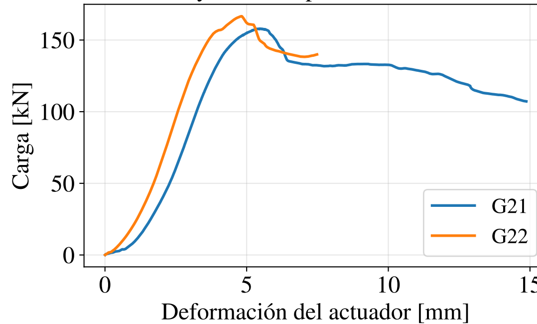
Ensayos de compresión: Guadua 2
