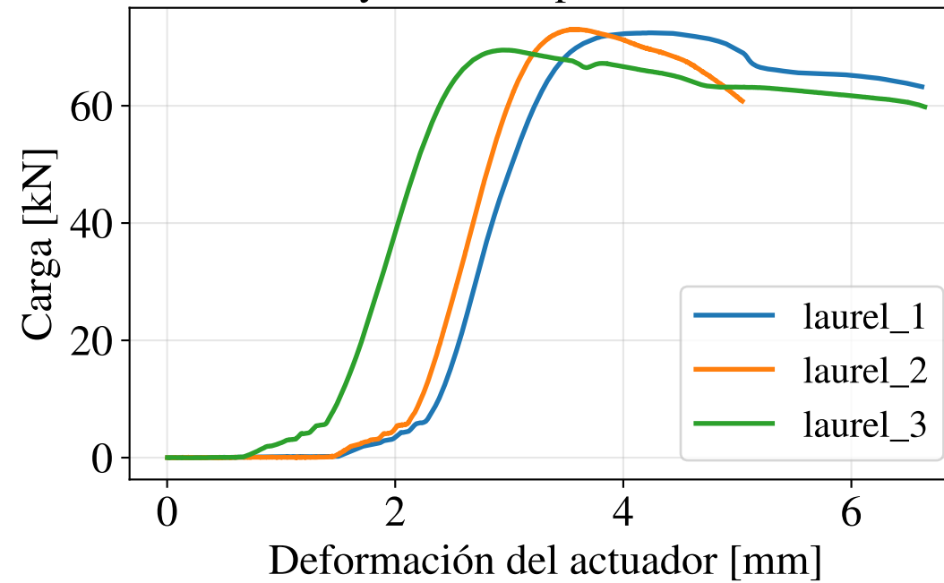
Ensayos de compresión: Laurel
