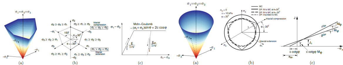
(a) Criterio de Mohr-Coulomb.
