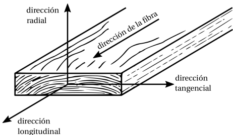
Figure: Direcciones de ortotropía de la madera.
