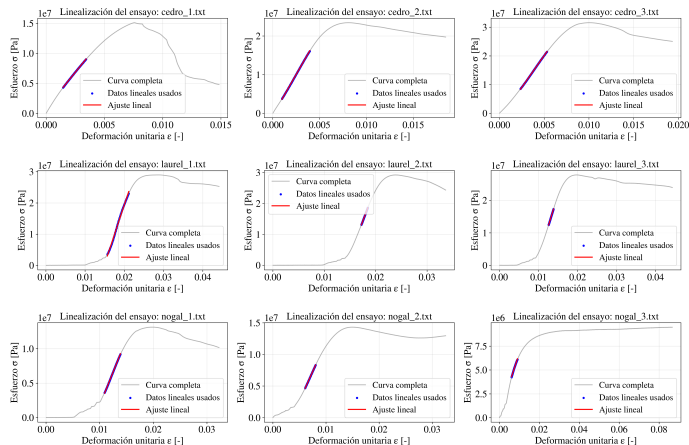
Figure: Autoría propia. Ver: https://github.com/michaelherediaperez/procesamiento-datos-ensayos-compresion .
