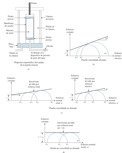
Figura 1.26 Prueba triaxial.
