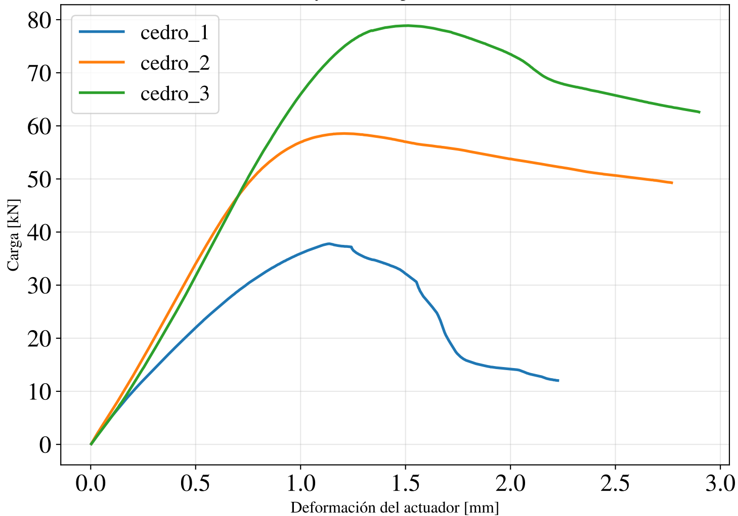
Ensayos de compresión: Cedro
