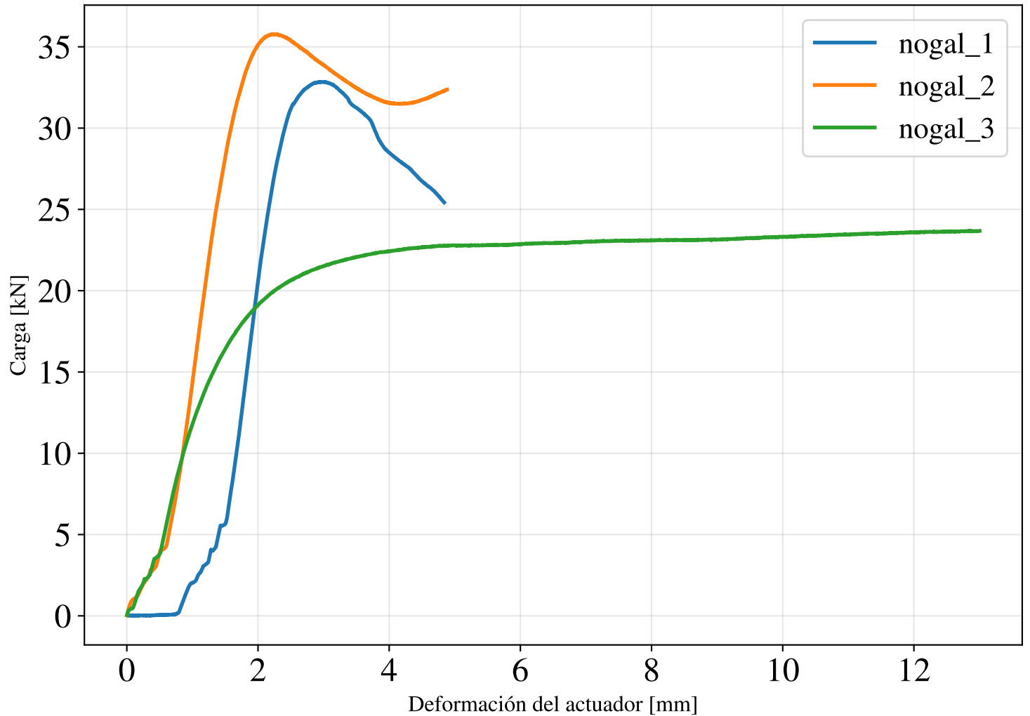
Ensayos de compresión: Nogal
