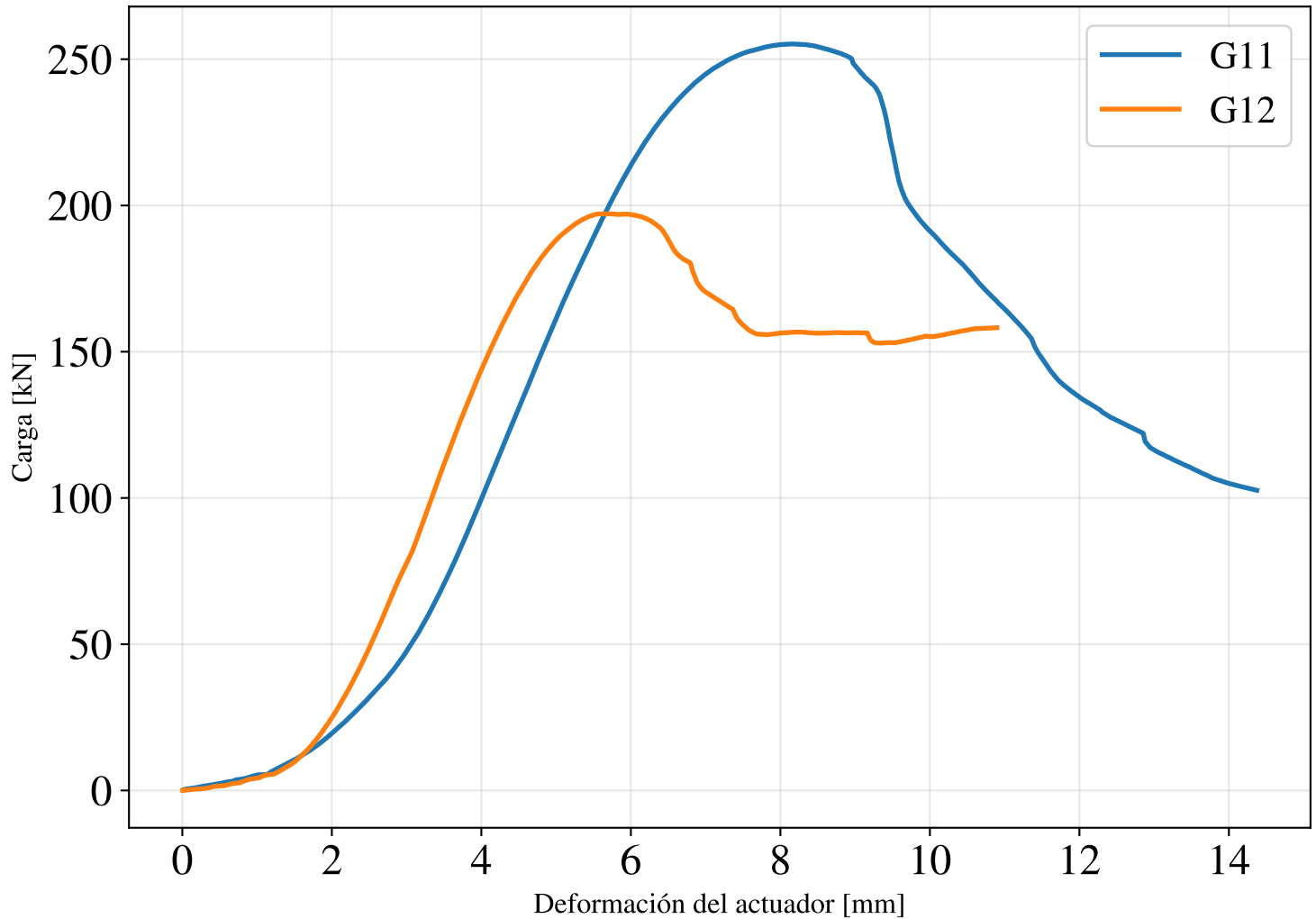
Ensayos de compresión: Guadua 1
