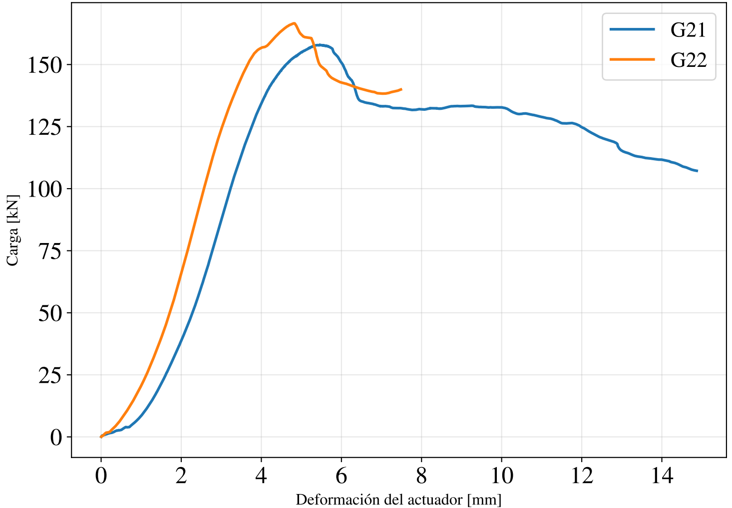
Ensayos de compresión: Guadua 2
