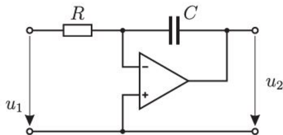
Abbildung 27: Schaltung eines Integrators [17]
