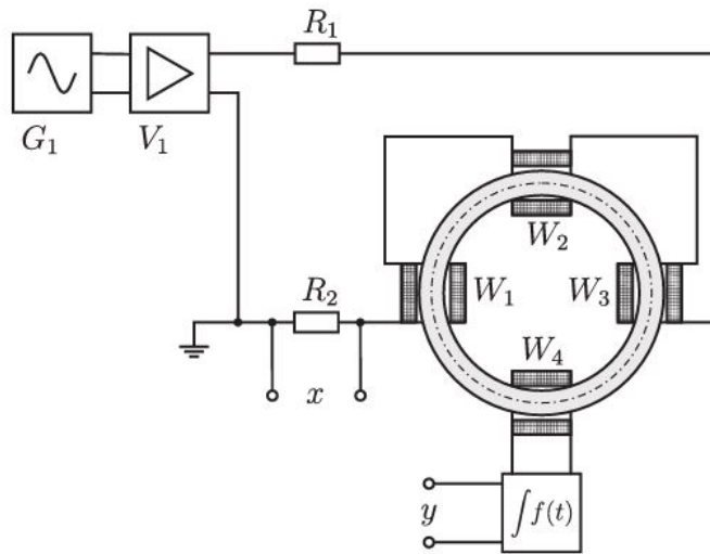
Abbildung 28: Messaufbau zur Messung der Hystereseschleife [17]
