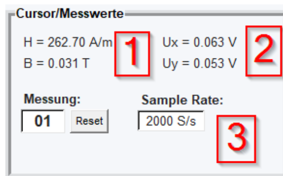
Abbildung 23: Cursor und Messwerte
