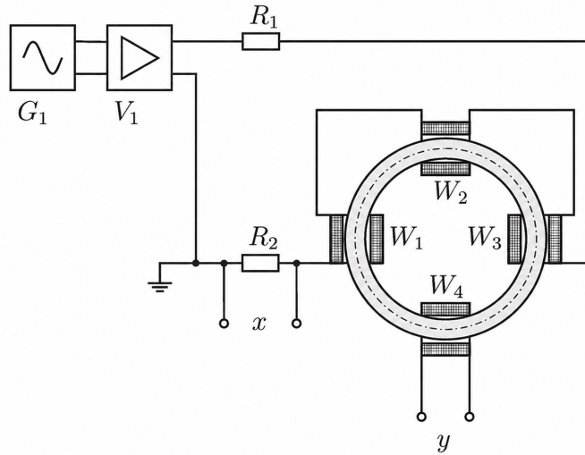
Abbildung 29: Messaufbau differentielle Permeabilität \mu_{\text{diff}} [17]
