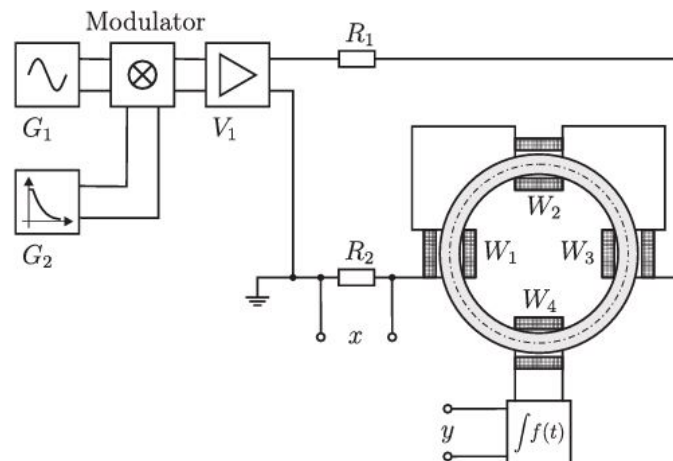
Abbildung 30: Messaufbau Entmagnetisierungskurve [17]
