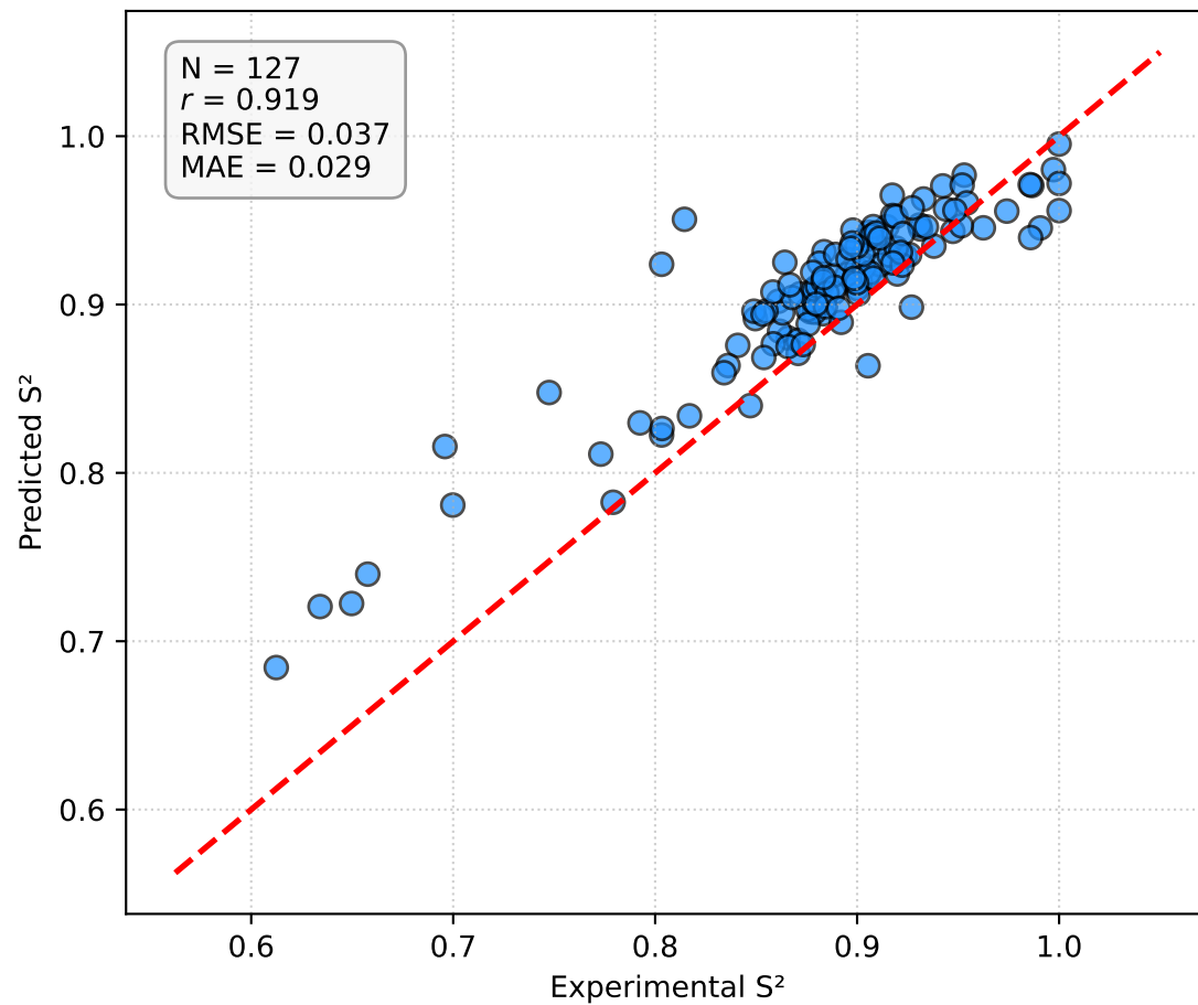
Order Parameters ( S^2 )
