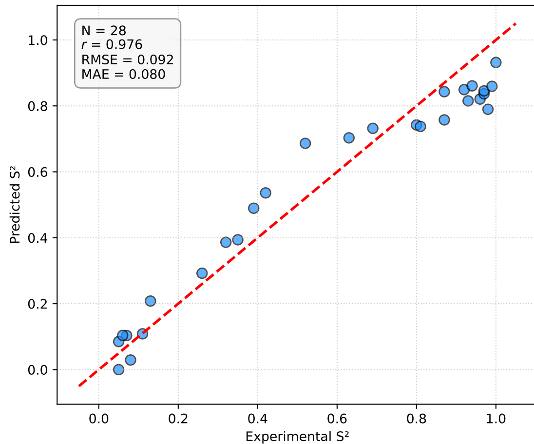
Order Parameters ( S^2 )
