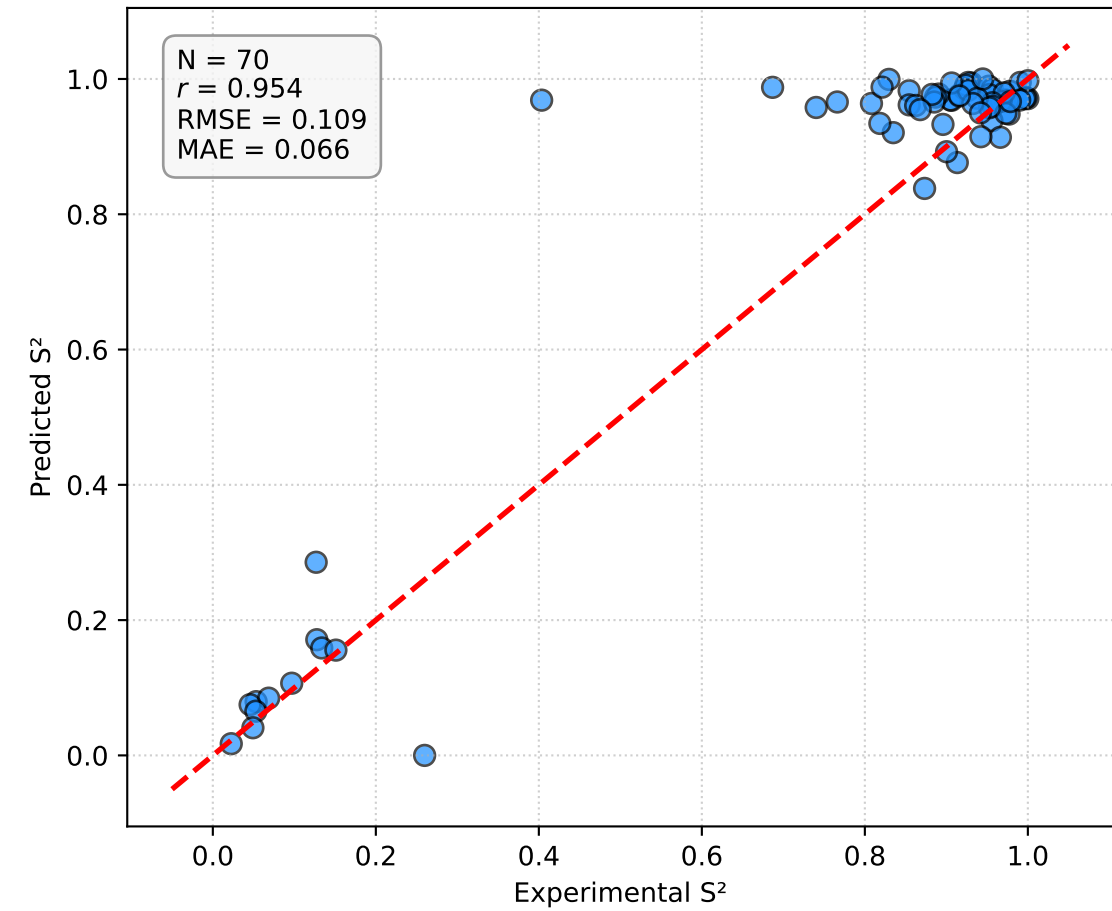
Order Parameters ( S^2 )
