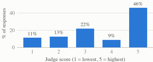
Gemma 4 26B ( M = 3.65 , SD = 1.44 , N = 153,569 )
