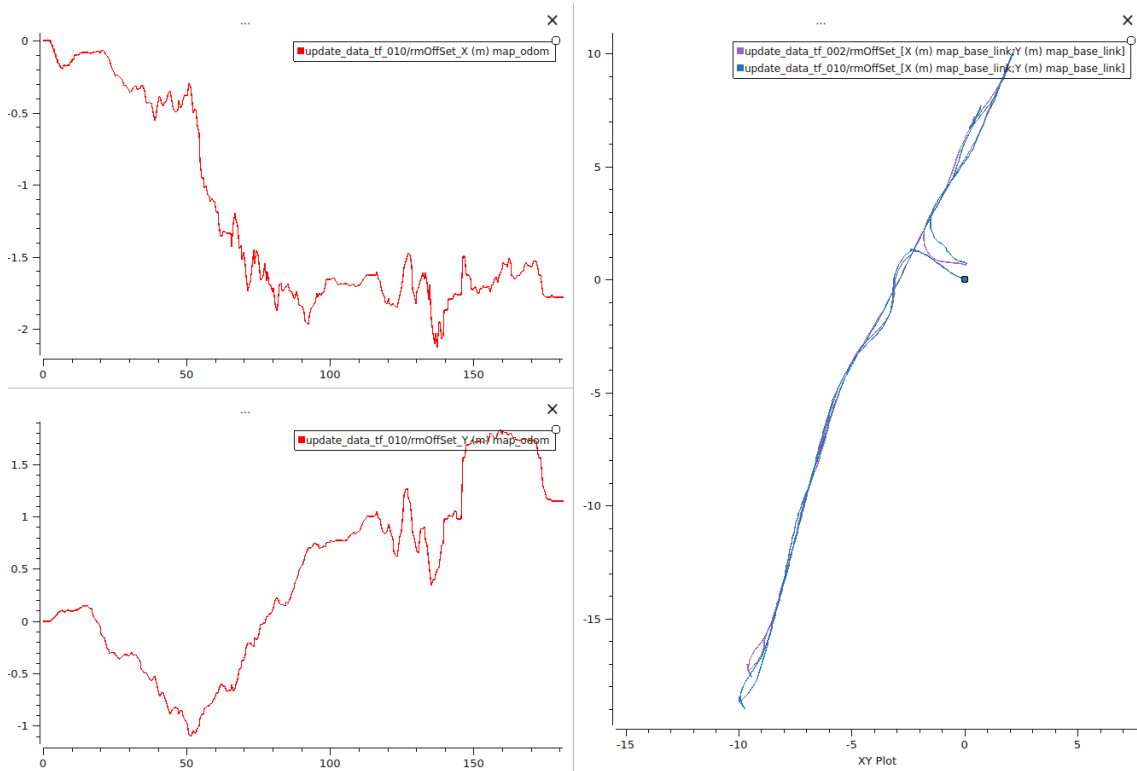
Figure 12.18: best result mini data plotted
