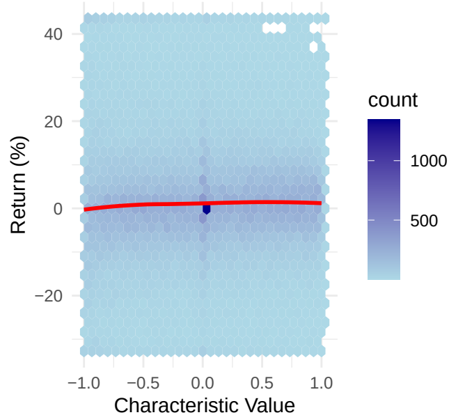
rank_dolvol
