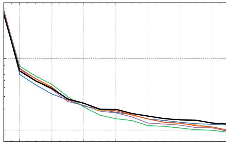
Gaps, (2000, 30)
