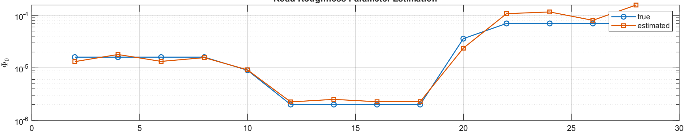
Road Roughness Parameter Estimation
