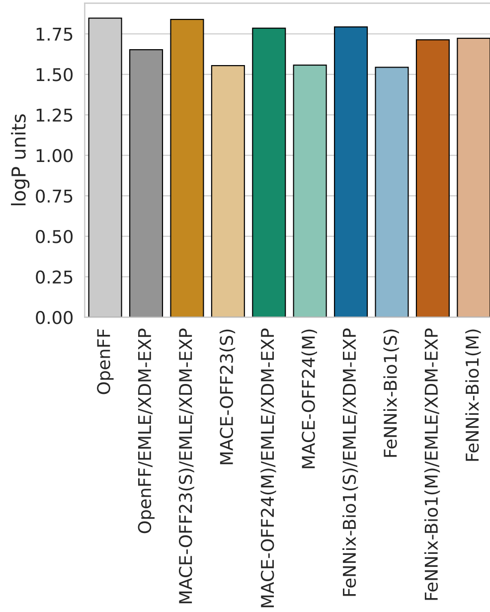
MAE
