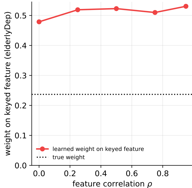
Parameter harm: invariant to correlation
