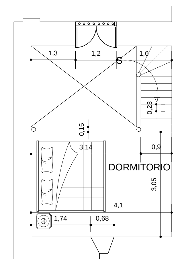
DETALLE MEZANINE DE HABITACIÓN 1 Esc. 1:50 AREA: 36,8898
