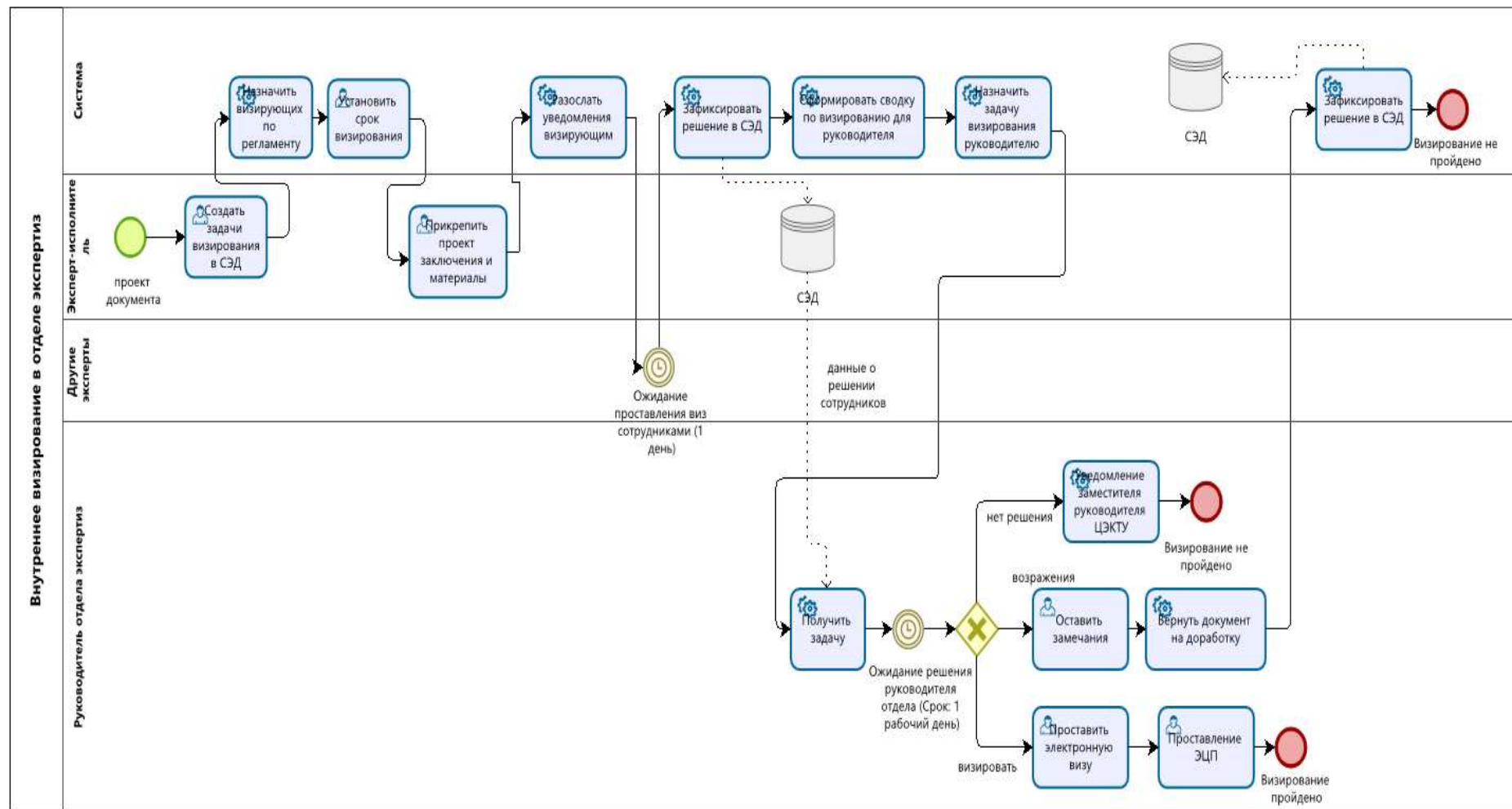
Рисунок 2.14 –Подпроцесс «Внутреннее визирование в отделе экспертиз»
