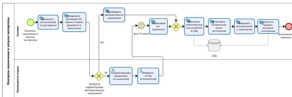
Рисунок 2.12 –Подпроцесс «Контроль назначения и запуск экспертизы»
