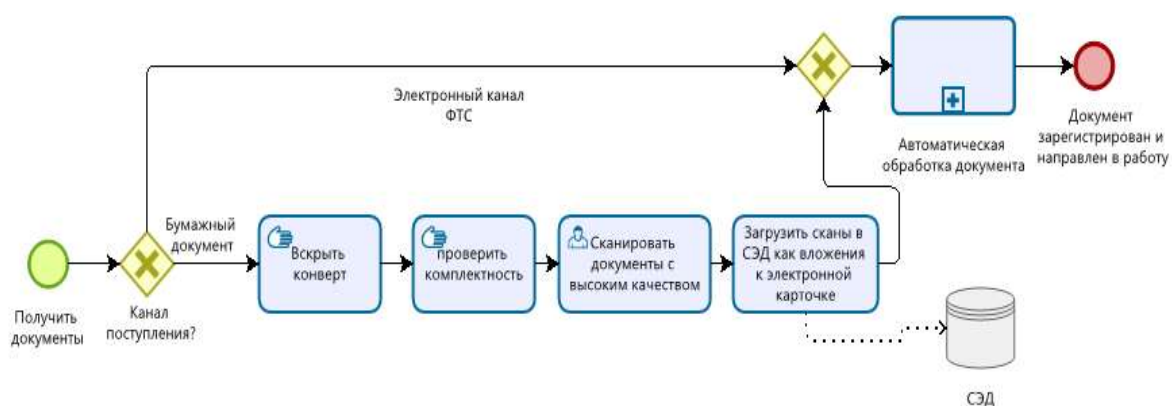
Рисунок 2.9 –Подпроцесс «Первичная обработка входящего документа»
