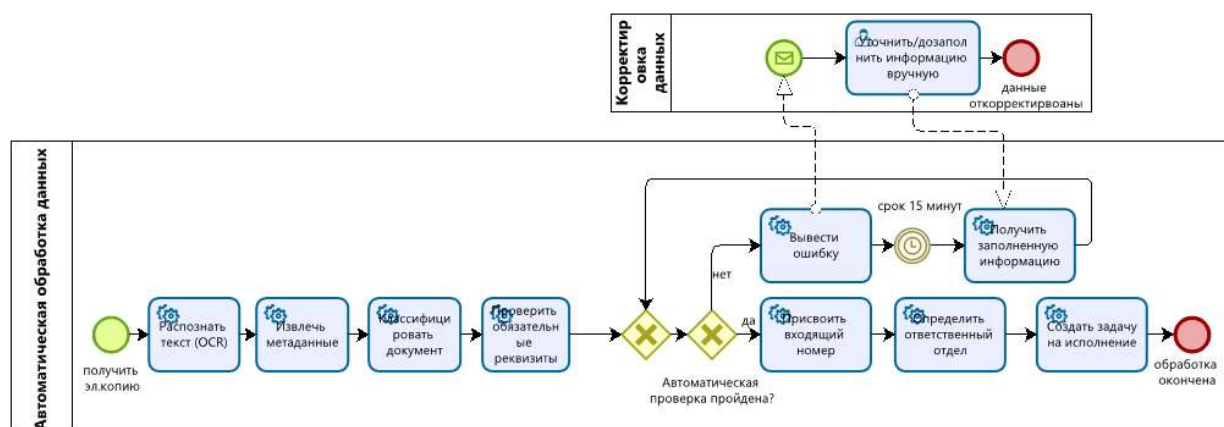
Рисунок 2.11 – Подпроцесс «Автоматическая обработка документа»
