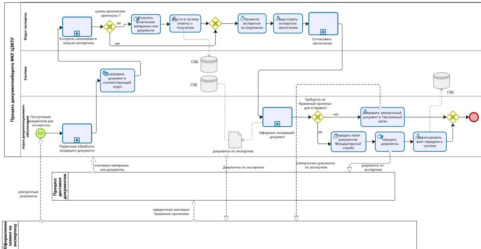
Рисунок 2.9 – Модель «to-be» в нотации BPMN. Процесс документооборота ФКУ «ЦЭКТУ»
