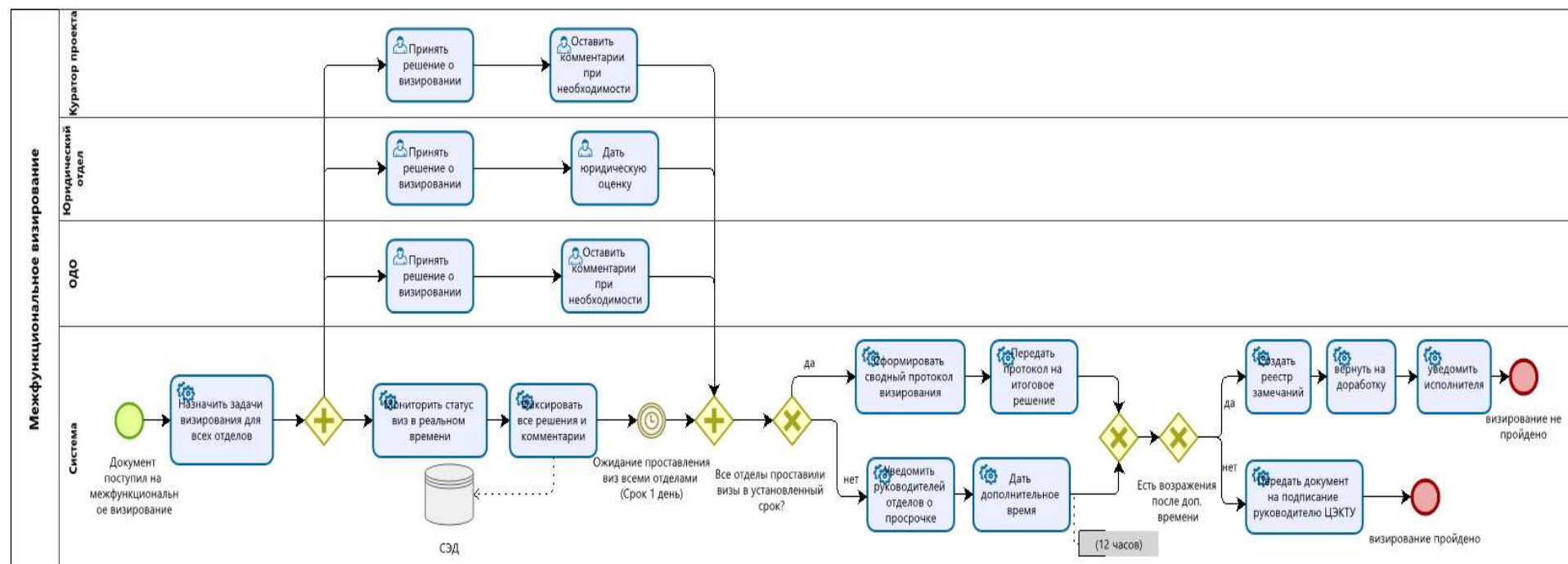
Рисунок 2.15 –Подпроцесс «Межфункциональное визирование»
