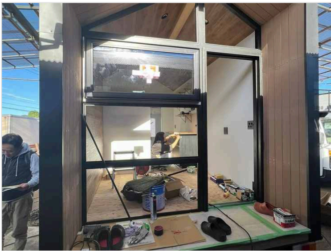
黒い骨組みに切妻屋根。中では造作が進んでいた
